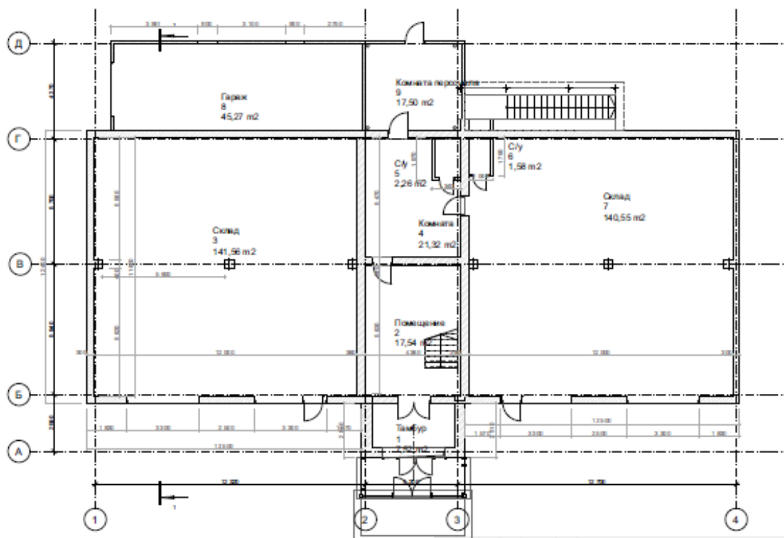
План 1-го этажа после реконструкции
