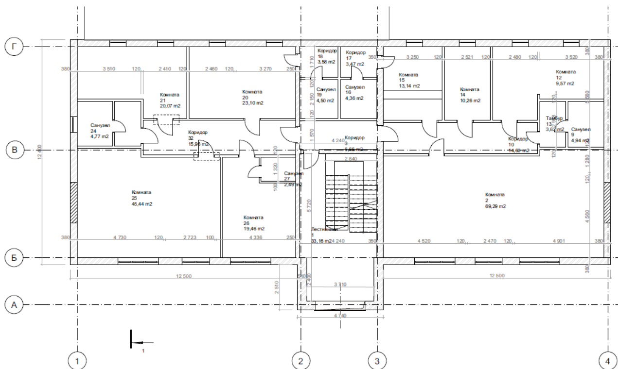
План 2-го этажа после реконструкции
