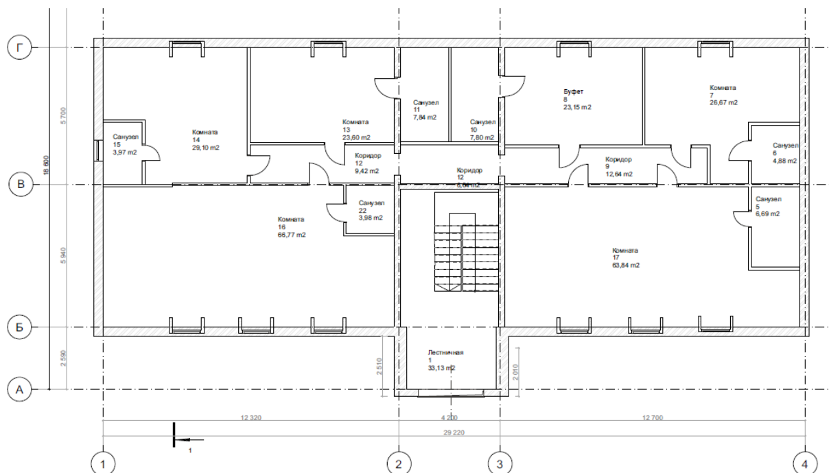
План мансардного этажа после реконструкции
