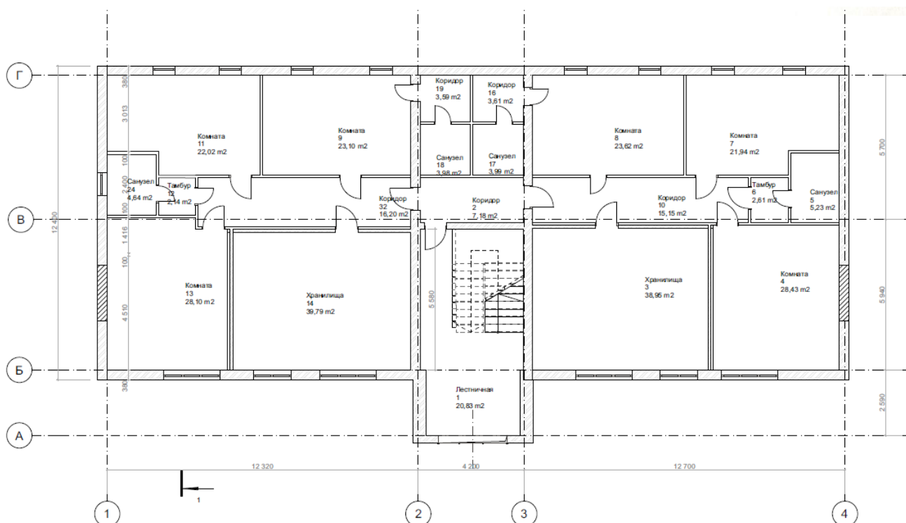
План 3-го этажа после реконструкции
