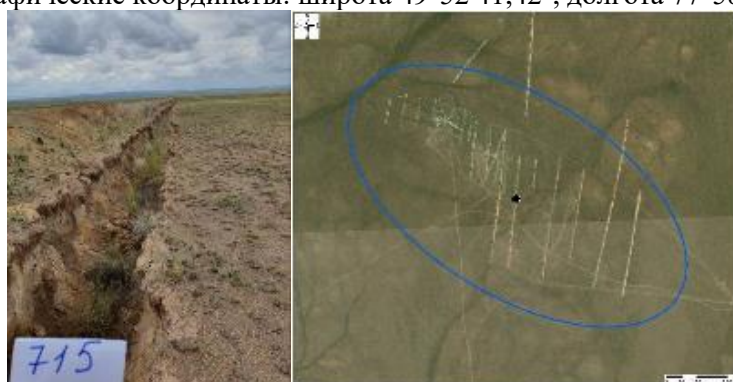
Рисунок 1492 - Объект 715. Сеть траншей 200x1x1,5, у начала траншей наклонные скважины (Географические координаты: широта 50°0'2,682", долгота 77°55'32,719")
