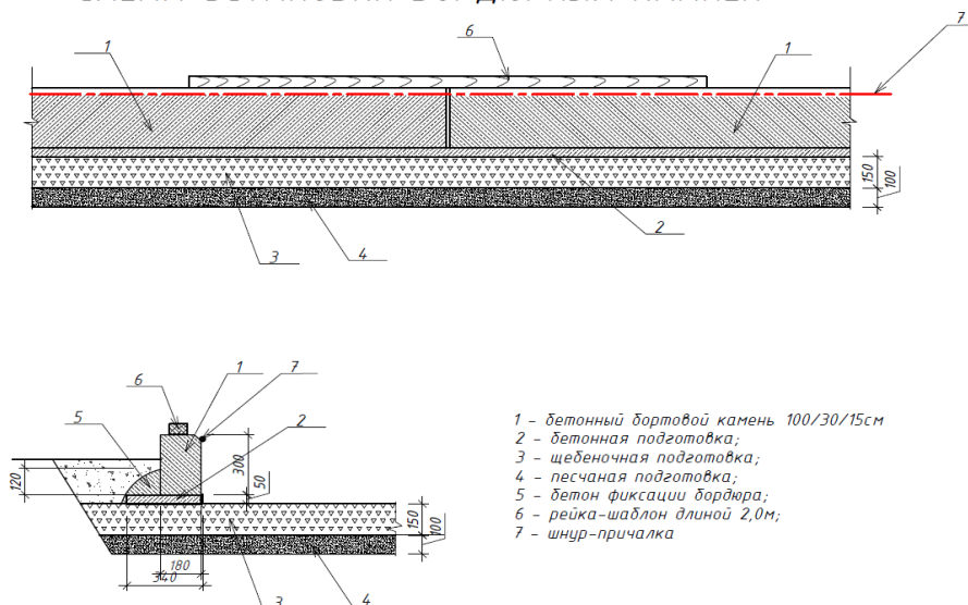
СХЕМА УСТАНОВКИ БОРДЮРНЫХ КАМНЕЙ
