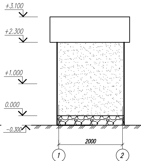
Фасад 1-2
