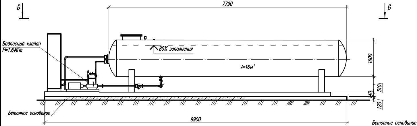
ВИД А-А
