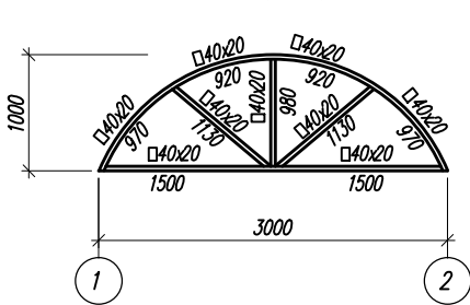
Геометрическая схема фермы Ф-1
