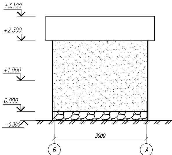
Фасад Б-А
