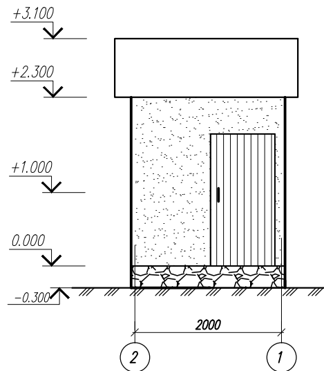
Фасад 2-1
