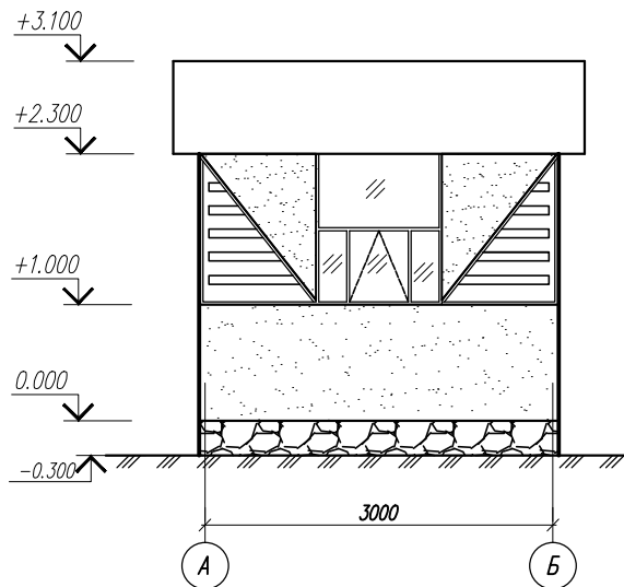
Фасад А-Б
