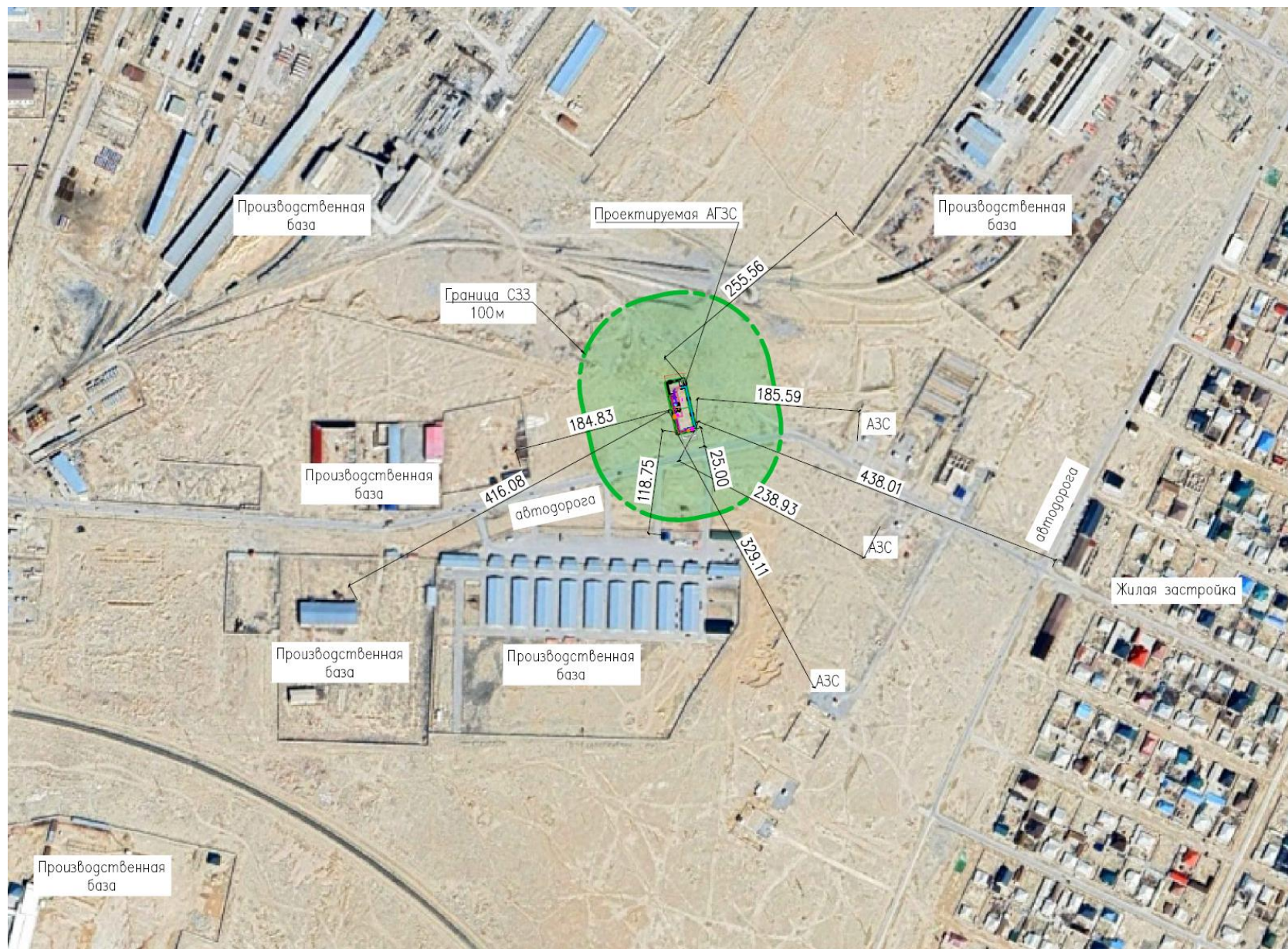
Рис. 1.1. Ситуационная карта расположение АГЗС
