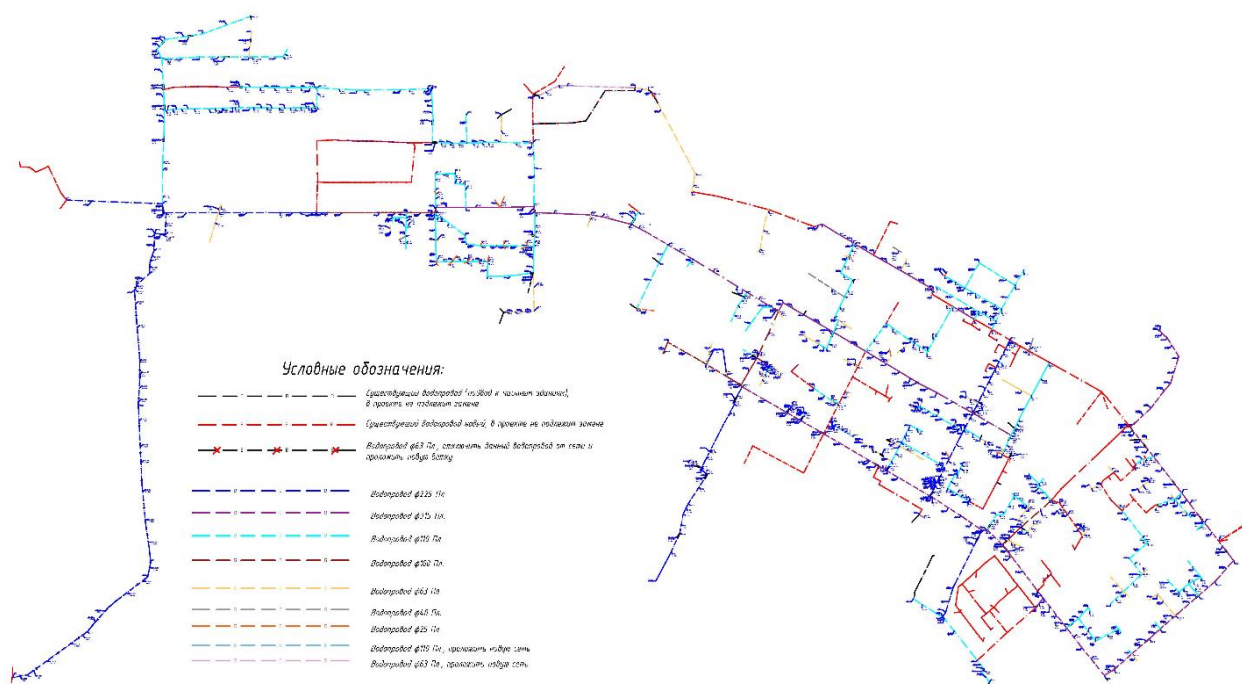
Рис. 1.2 – Схема прокладки инженерных сетей водоснабжения
