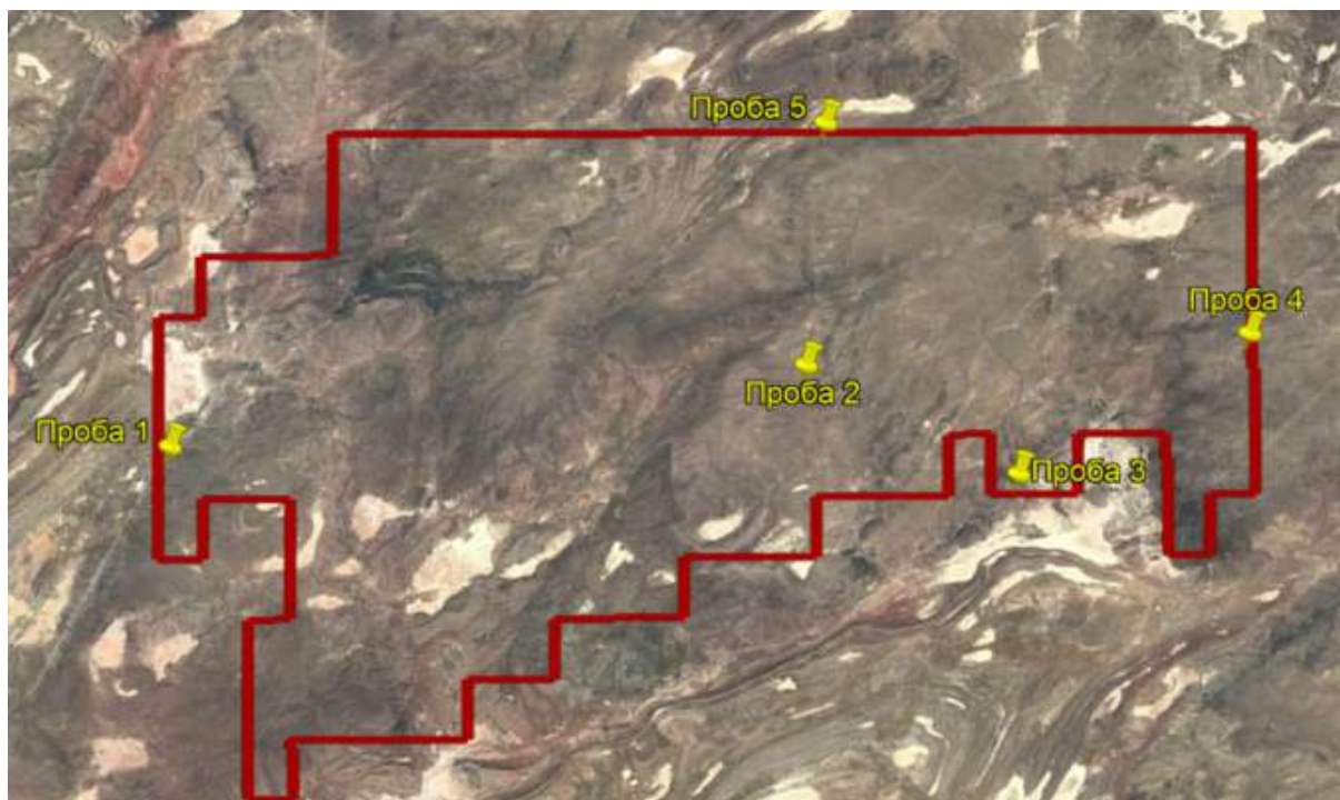
Рисунок 2.2 – Карта-схема с указанием точек фоновых концентраций
