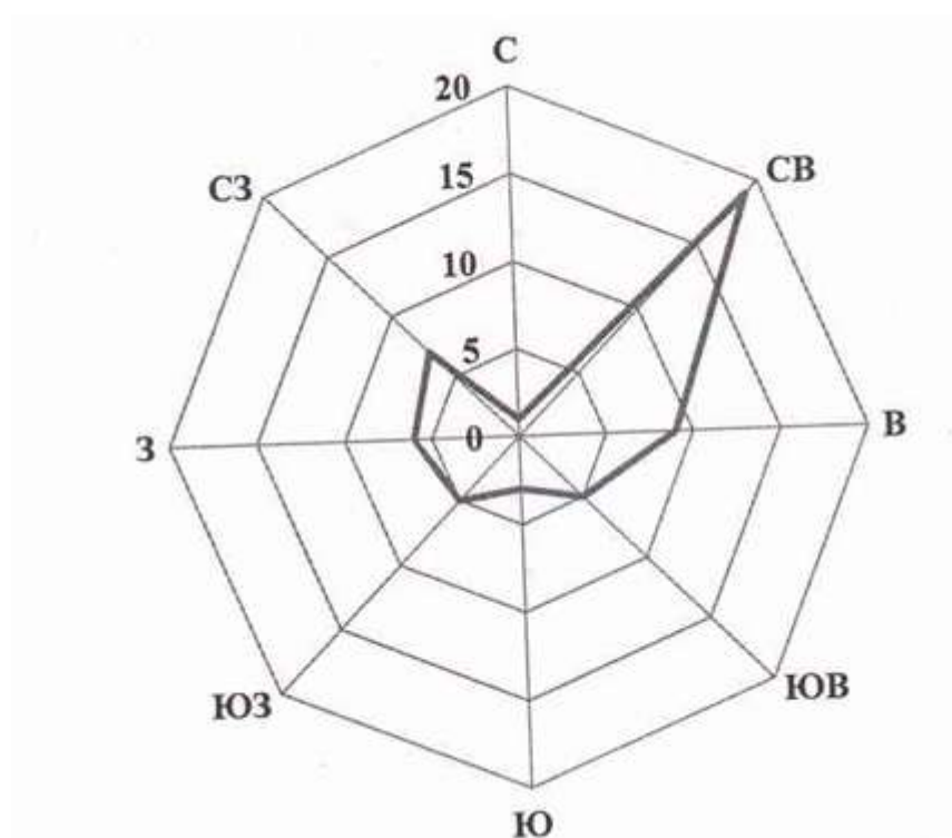
Рисунок 2.1 – Среднегодовая роза ветров района расположения рассматриваемой территории
