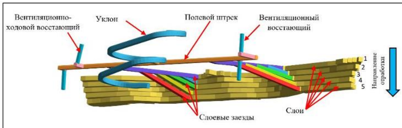
Рисунок 4.4 – Типовая схема подготовки блока
