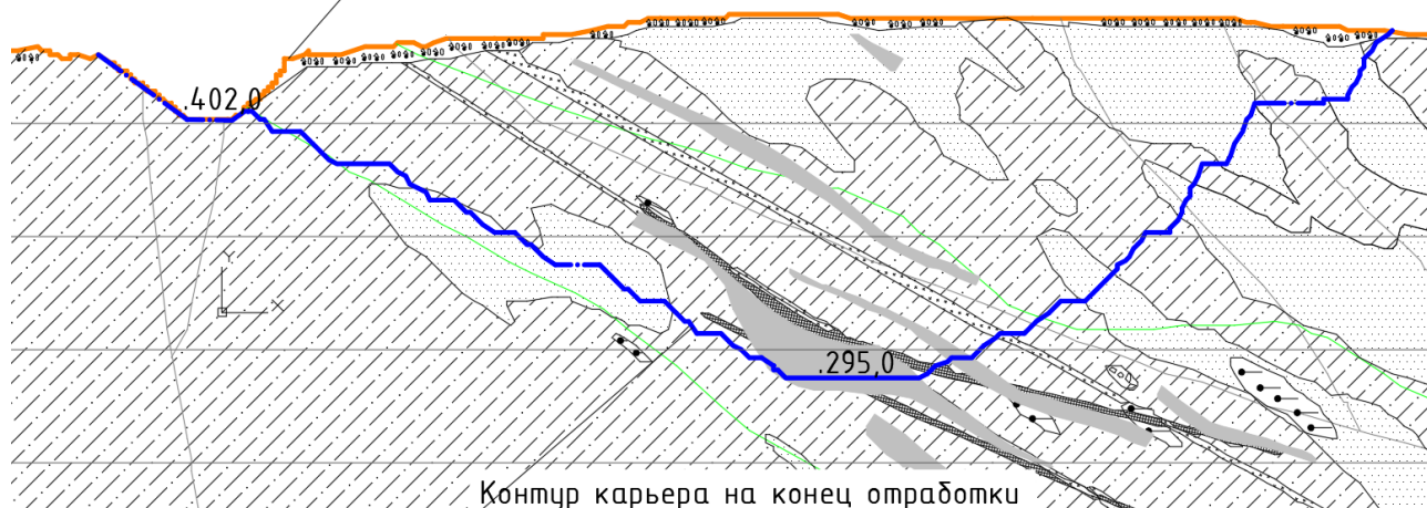
Рисунок 5.3.3. Геологический разрез по линии 4
