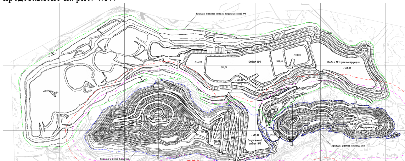
Рисунок 4.17. План расположения отвалов на конец отработки карьеров
