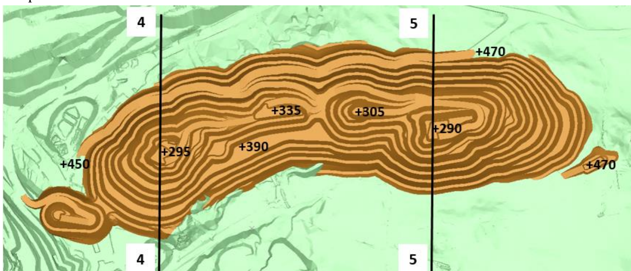
Рисунок 5.3.2. Трехмерный вид конструктивного контура Карьера № 2 на конец отработки Контур карьера на 01.01.2025 года
