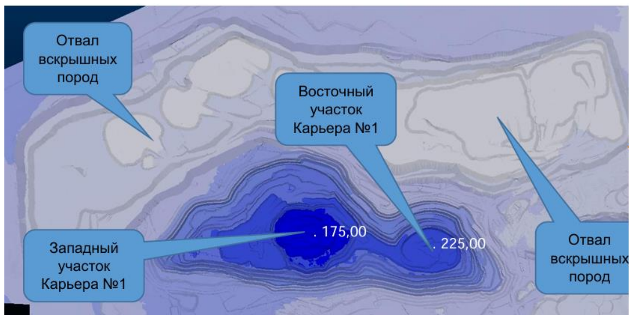
Рисунок 4.6.1. Фактическое положение горных (Карьер № 1) и отвалных (Отвал № 1) работ по состоянию на 01.01.2025 по Рудной зоне 1
