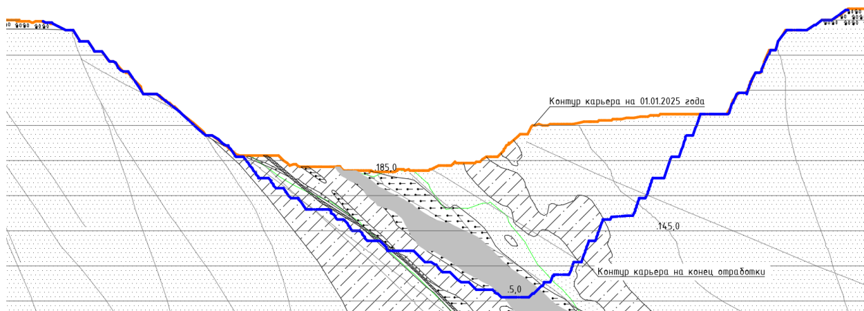
Рисунок 5.3.1. План и разрез А-А карьера № 1 на 2029 год
