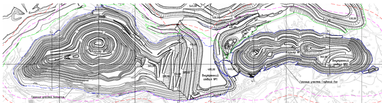
Рисунок 4.6.2. План карьеров на конец отработки
