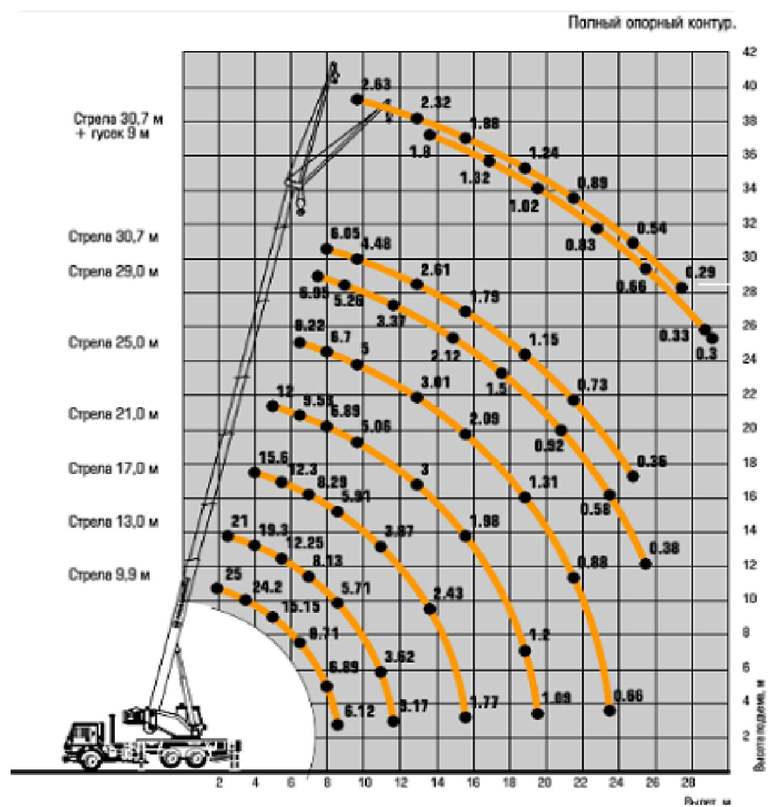
Автомобильный кран КС-45717К-1Р
