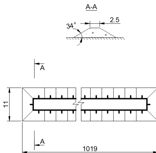
Рисунок 5 - План оградительной дамбы (борт)
