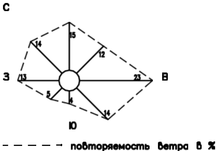
Рис. 1.3 Роза ветров
