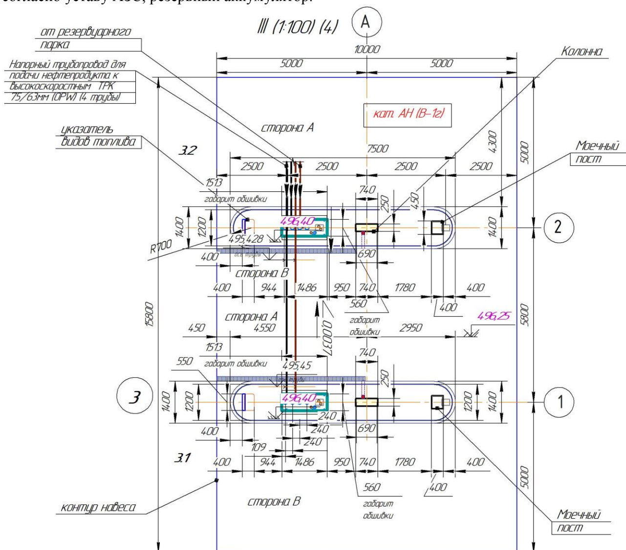
Рисунок 3.6 - ТПК Tokheim, Quantum Quantum ML 2-4-2 VHS FHR Р. Общий вид
