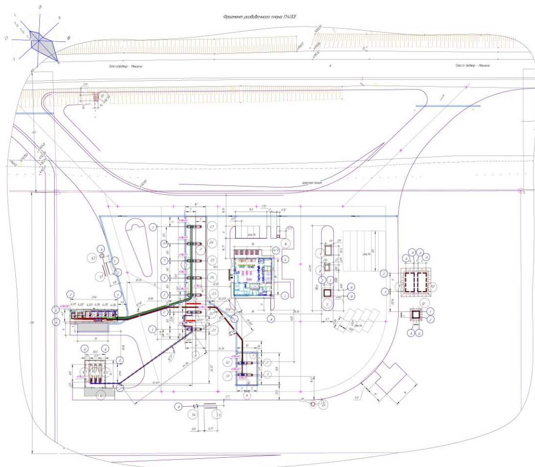
Рисунок 3.1 АЗС-АГЗС - Ситуационный план (засыпка условно не показана)
