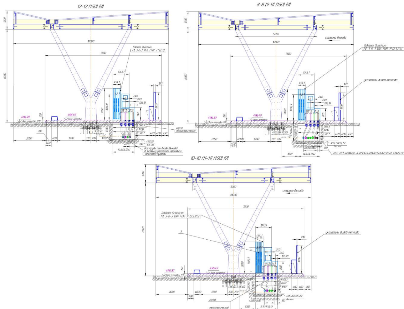
Рисунок 3.5 - Tokheim Quantum ML 3-6-3 VR4 FHR P. Разрезы
