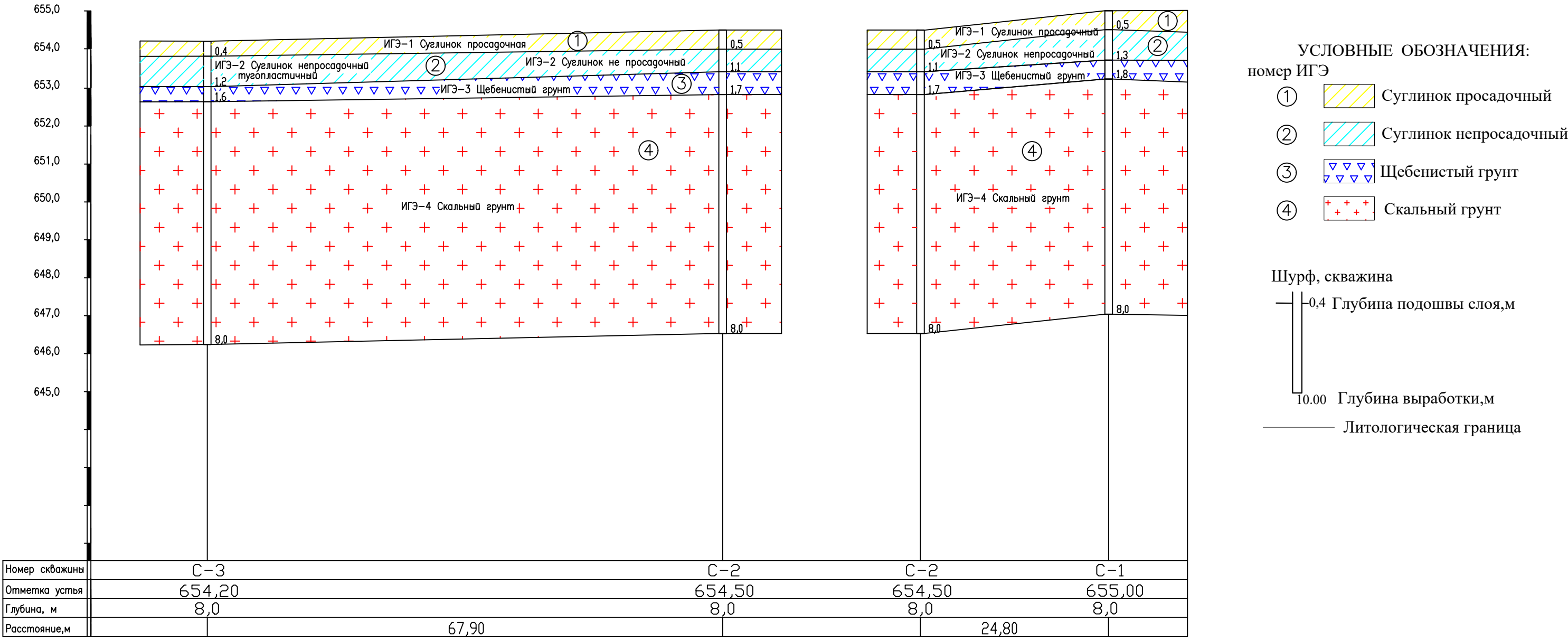
Инженерно-геологический разрез по линии I-I
