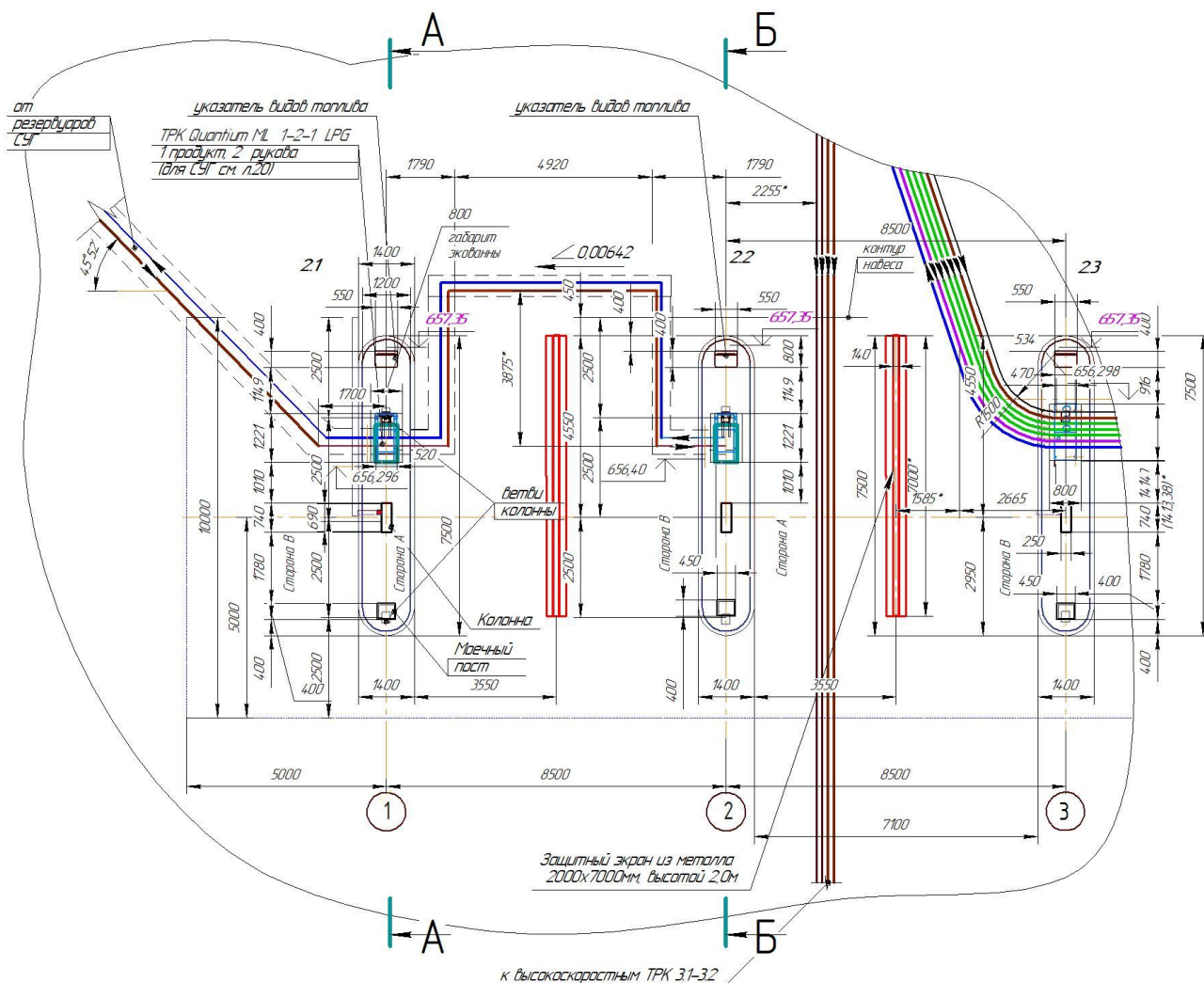
Рисунок 3.12 - ГРК Tokheim Quantum ML 1-2-1 LPG. Общий вид
