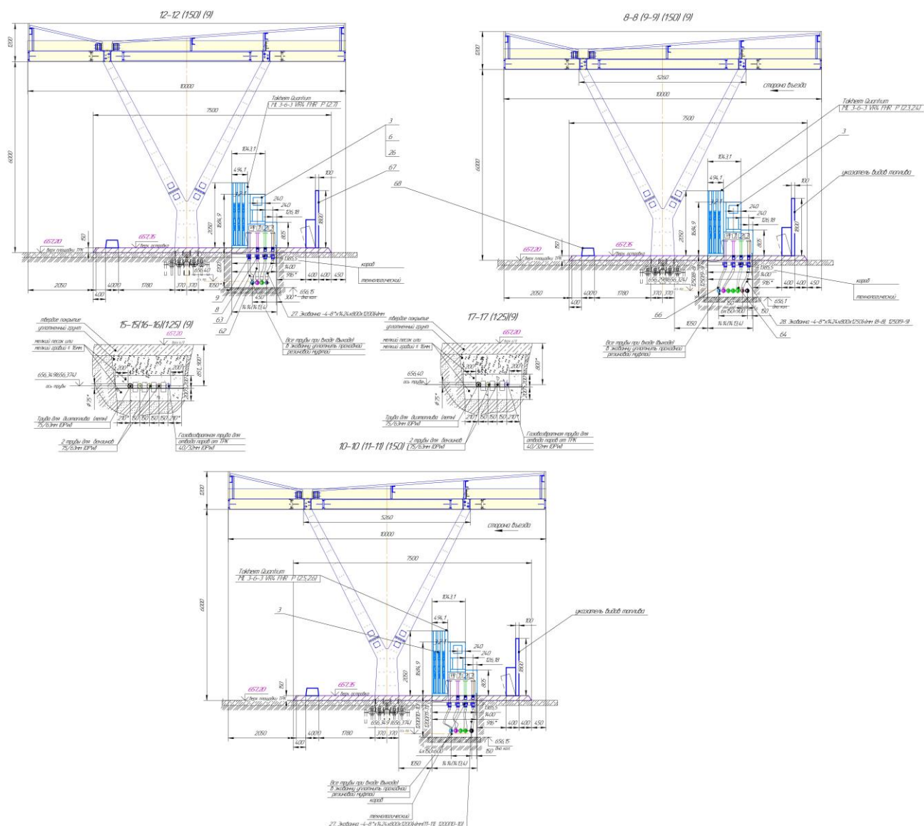
Рисунок 3.5 - Tokheim Quantum ML 3-6-3 VR4 FHR P. Разрезы Техническая характеристика ТРК Tokheim, Quantum ML 2-4-2 VHS FHR P Тип-Tokheim, Quantum ML 2-4-2 VHS FHR P
