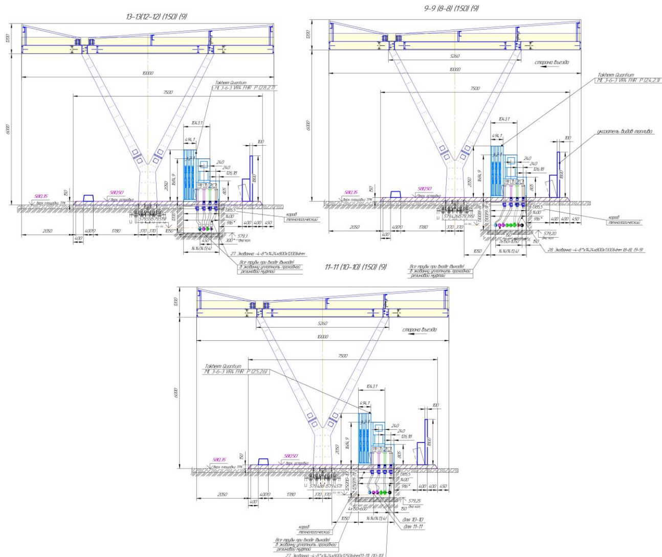
Рисунок 3.5 - Tokheim Quantum ML 3-6-3 VR4 FHR P. Разрезы
