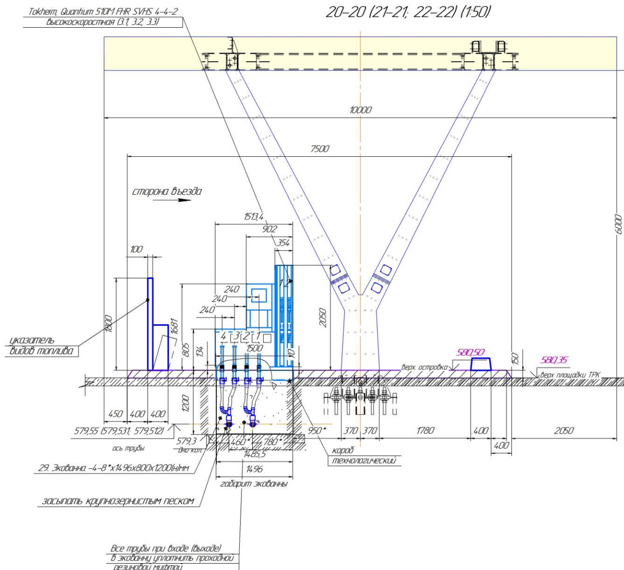
Рисунок 3.7 - ТРК Tokheim, Quantum ML 2-4-2 VHS FHR Р. Разрез Техническое обслуживание и проверка топливораздаточной колонки
