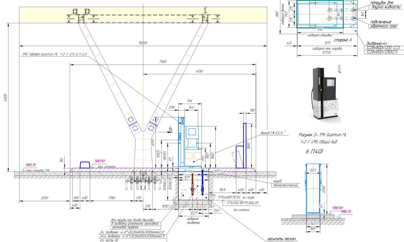
Рисунок 3.13 - ГПК Tokheim Quantum ML 1-2-1 LPG. Разрез
