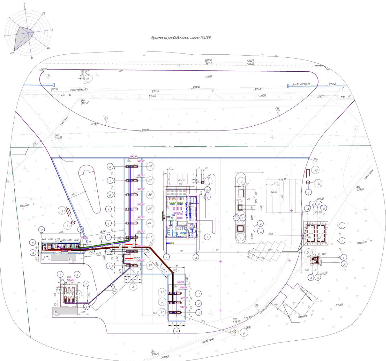
Рисунок 3.1 АЗС-АГЗС - Ситуационный план (засыпка условно не показана)
