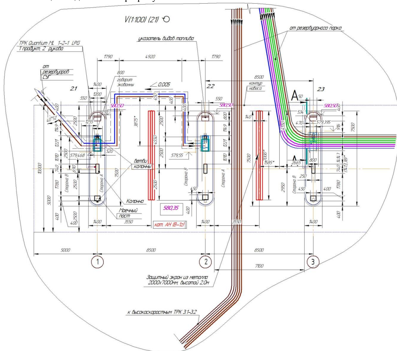
Рисунок 3.12 - ГРК Tokheim Quantum ML 1-2-1 LPG. Общий вид
