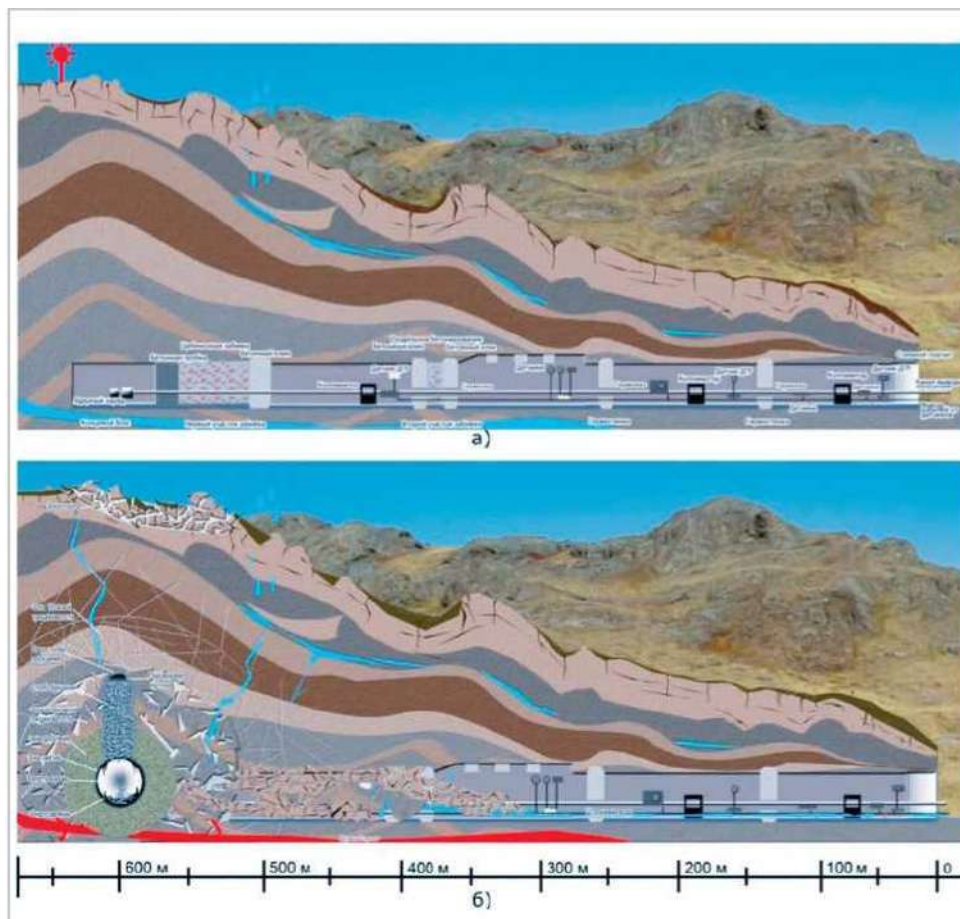
Рисунок 3.1.11 - Поперечный разрез штольни перед (а) и после (б) проведения испытания (схема)
