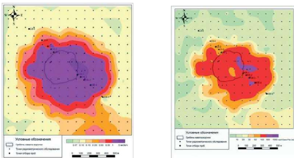
Рисунок 3.1.8 - Результаты радиоэкологического обследования на карте-схеме площадки «Сары-Узень»
