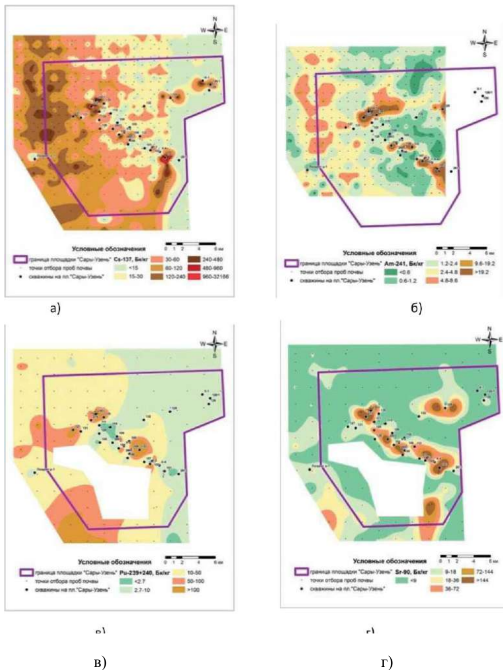
Рисунок 3.1.10 – Распределение радионуклидов на площадке «Сары-Узень» а) ^{137}\text{Cs} ; б) ^{241}\text{Am} ; в) ^{90}\text{Sr} ; г) ^{229+240}\text{Pu}
