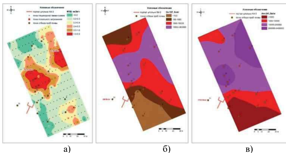
Рисунок 3.1.12 - Карты-схемы распределения МЭД (а), 137 Cs (б) и 241 Am (в) на территории одной из штолен площадки «Дегелен»
