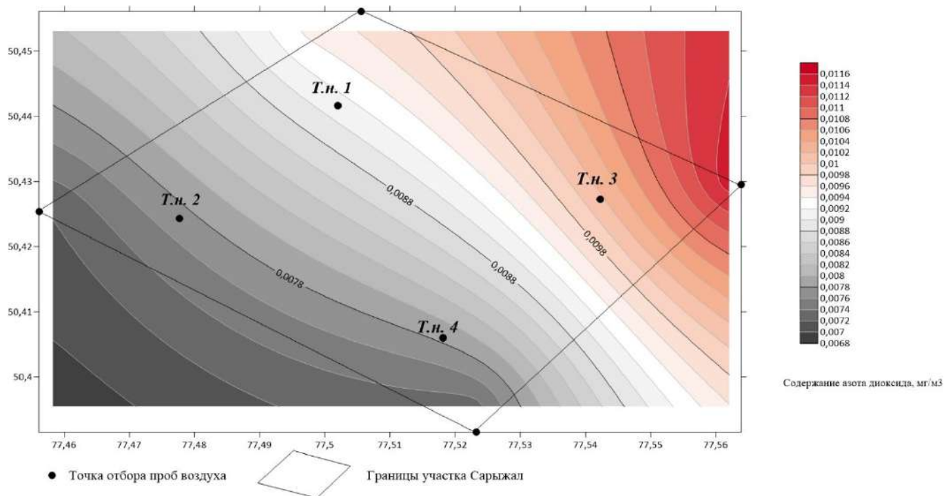
Рисунок 4.1.2 – Содержание азота диоксида в воздухе участка Сарыжал
