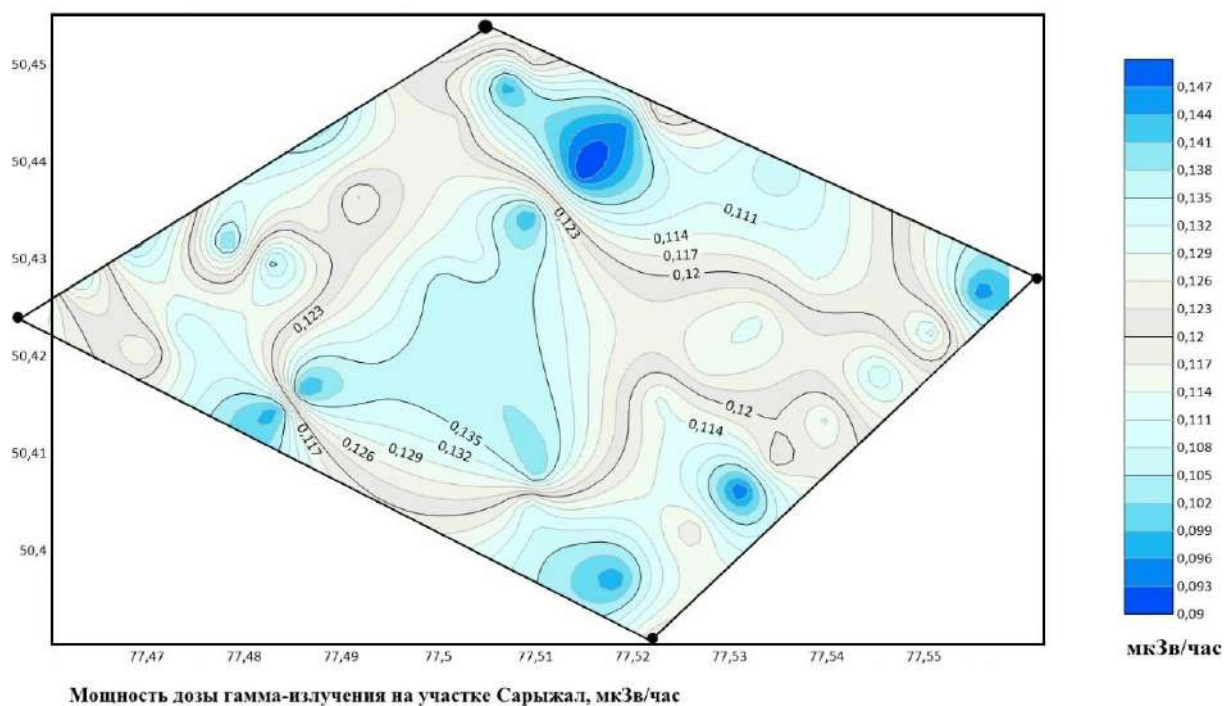
Рисунок 3.2.6 –Карта-схема распределения мощности дозы гамма-излучения на участке Сарыжал
