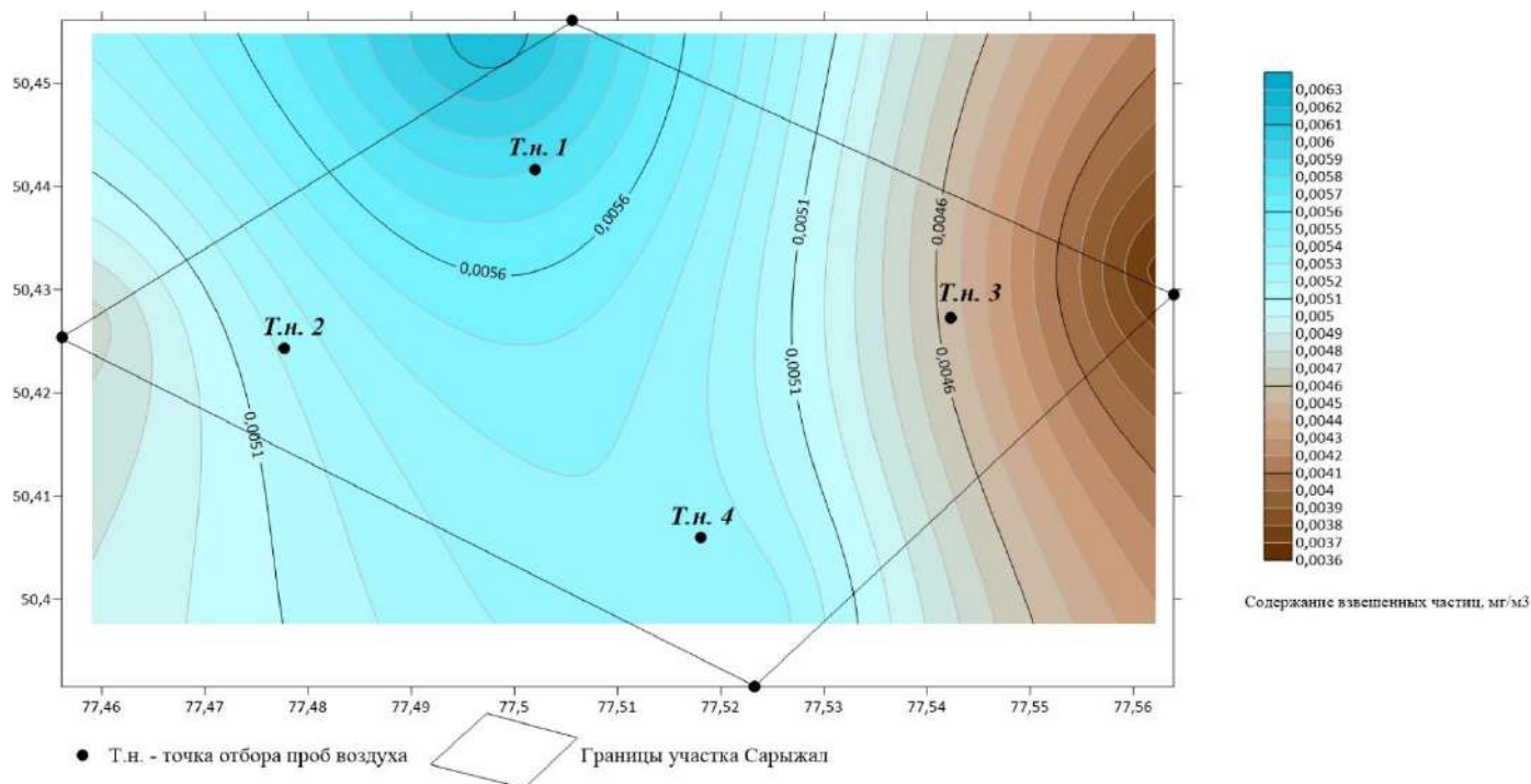
Рисунок 4.1.3 – Содержание взвешенных частиц в воздухе участка Сарыжал
