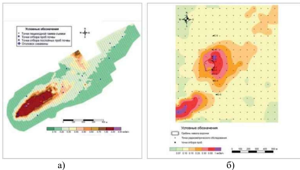
Рисунок 3.1.7 – Распределение МЭД на территории: а) скважина №215; б) скважина №1003
