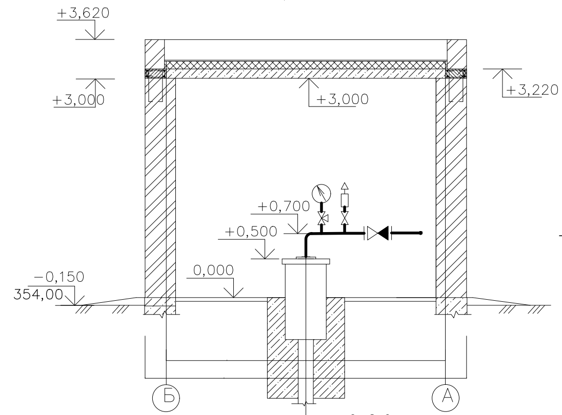
Разрез 1-1
