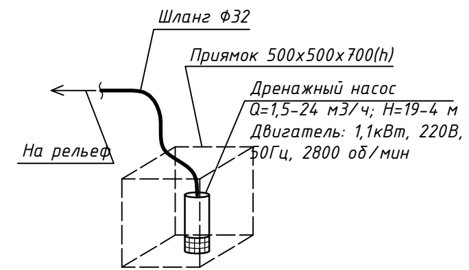
Схема системы КЗ
