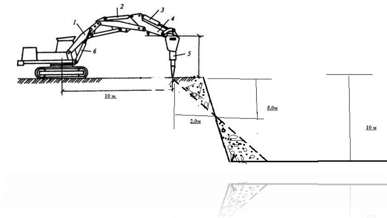
Рис. 10.1 Схема выполаживание бортов карьера.
