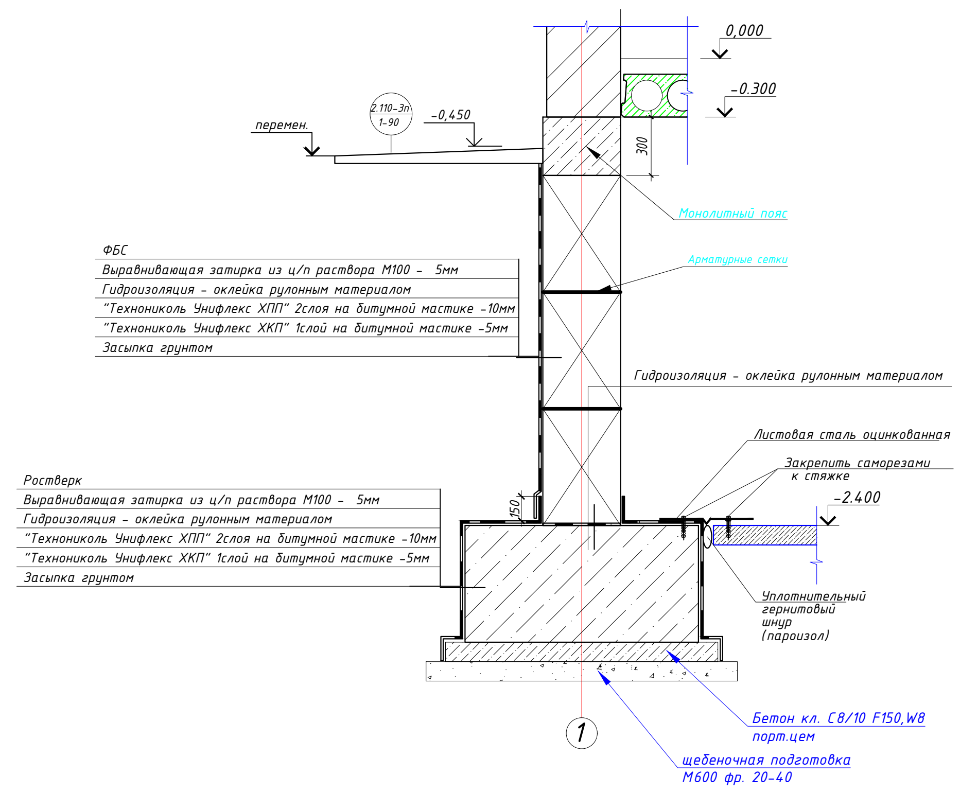
Узел примыкания наружной стены с фундаментом (гидроизоляция)
