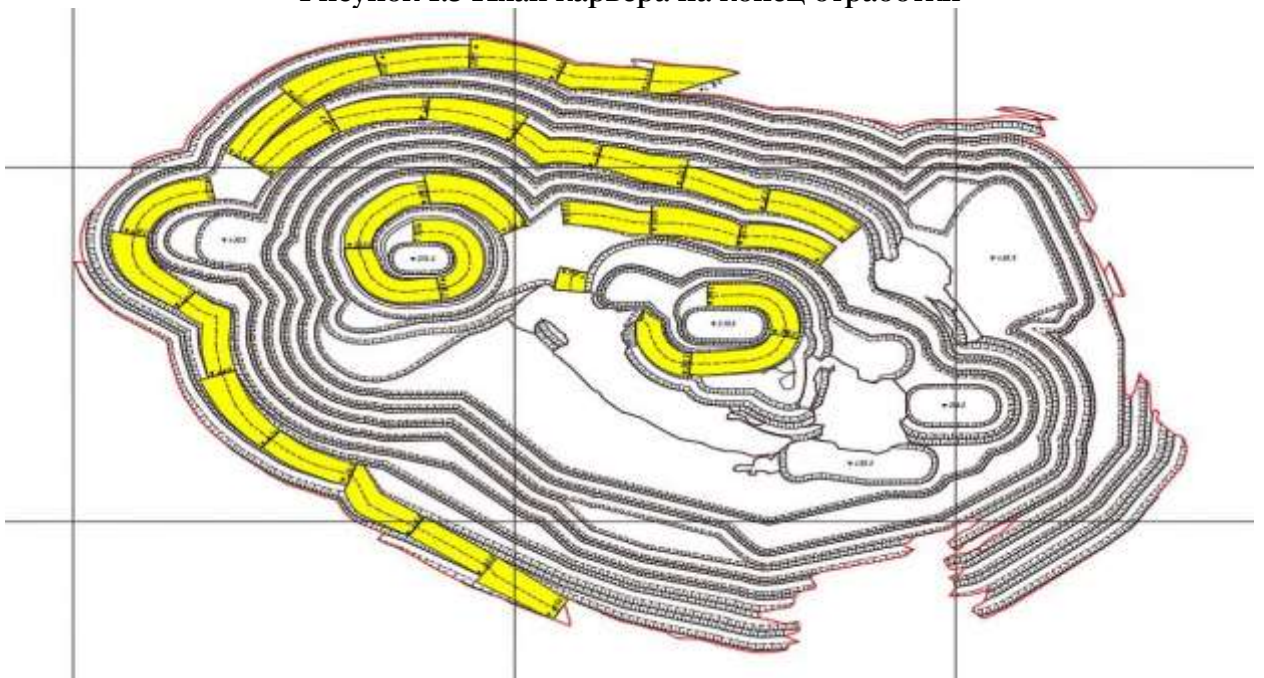
Рисунок 1.3 План карьера на конец отработки
