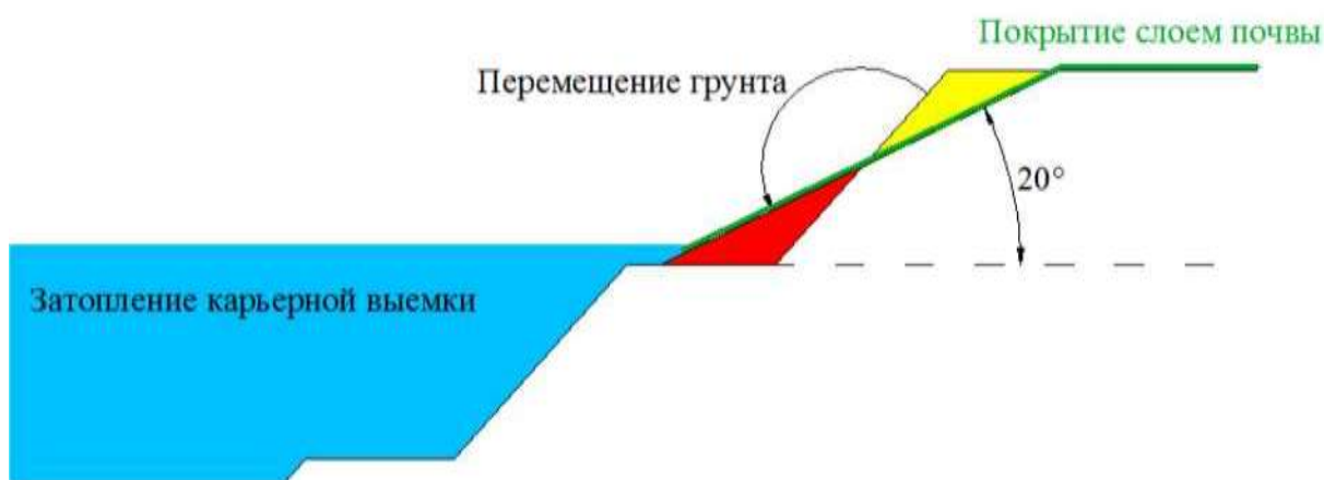
Рисунок 1.4 Схема ликвидации карьерной выработки
