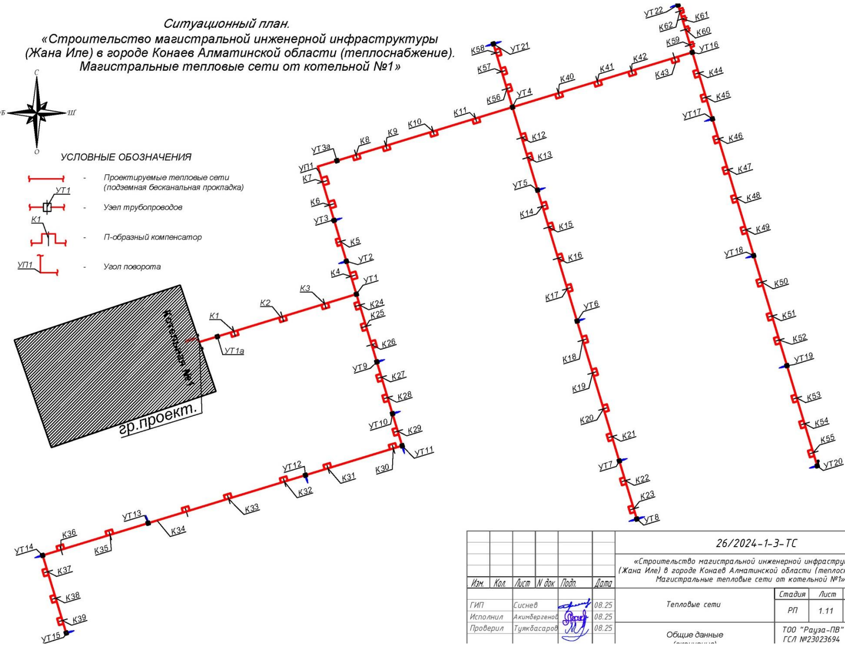
Рисунок 1 – Ситуационный план проектируемого объекта
