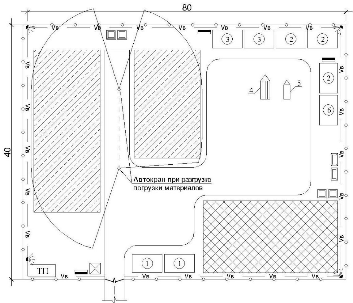
Рисунок 1 – Временный стройдвор
