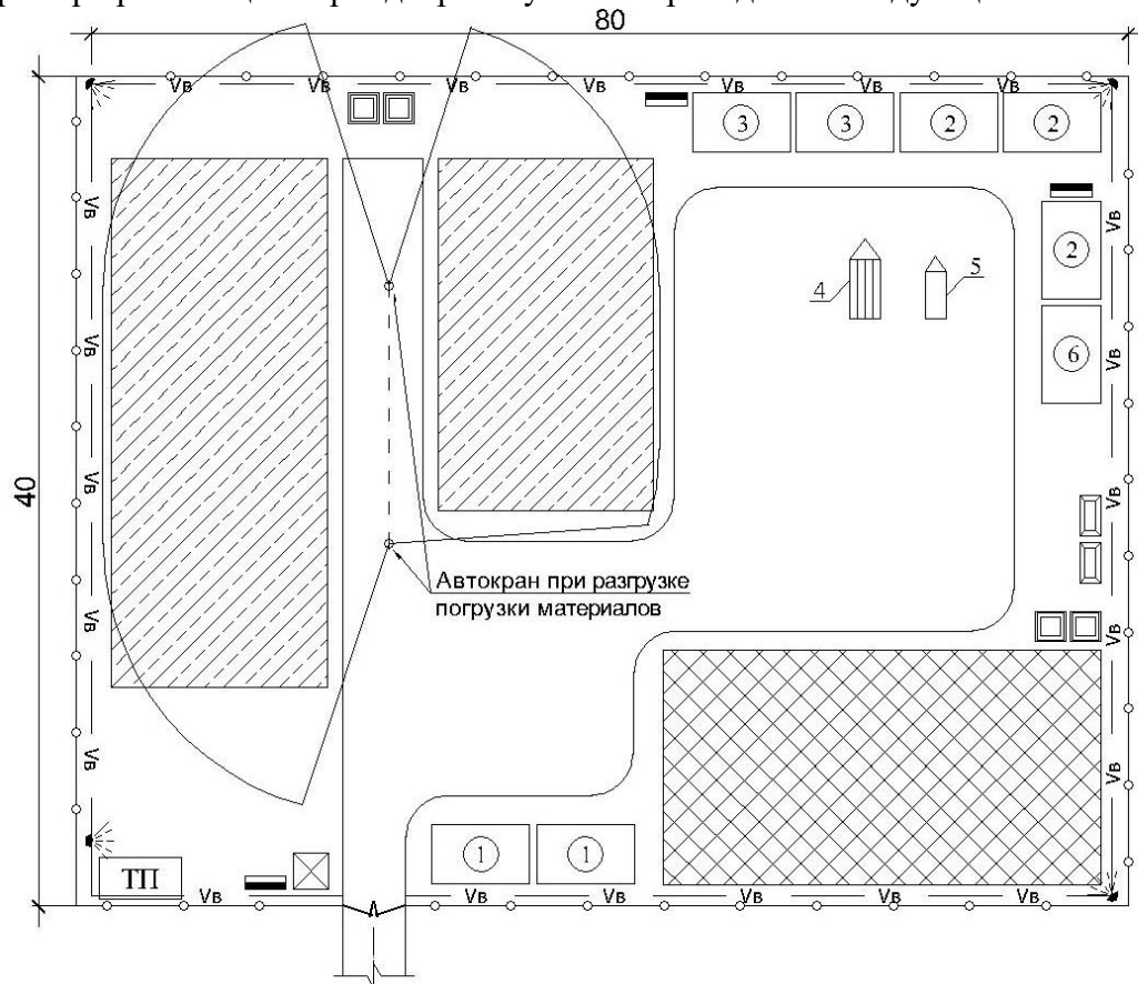
Рисунок – 2. Временный стройдвор
