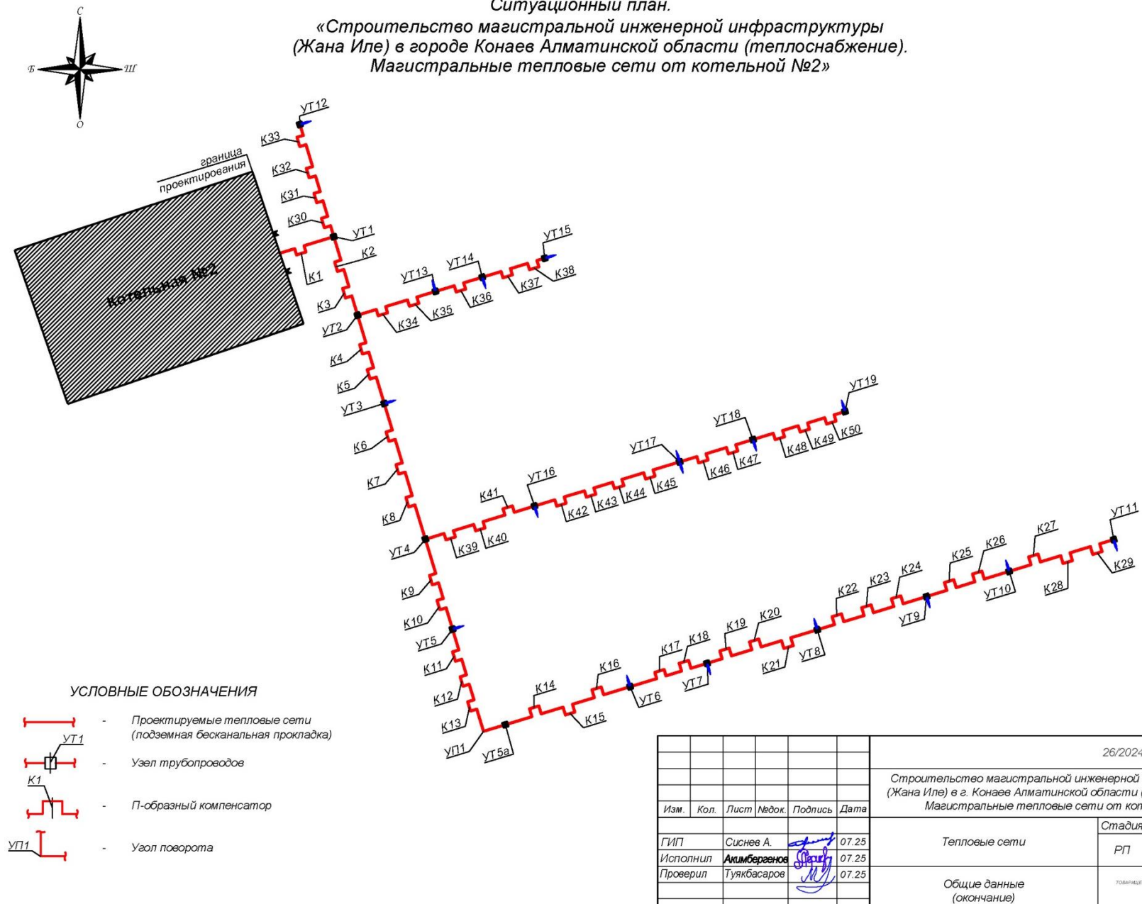
Рисунок 1 – Ситуационный план проектируемого объекта
