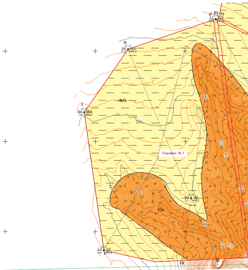
Рис.3.1 Схема геологического строения месторождения «Нура-2 (участок №1)»
