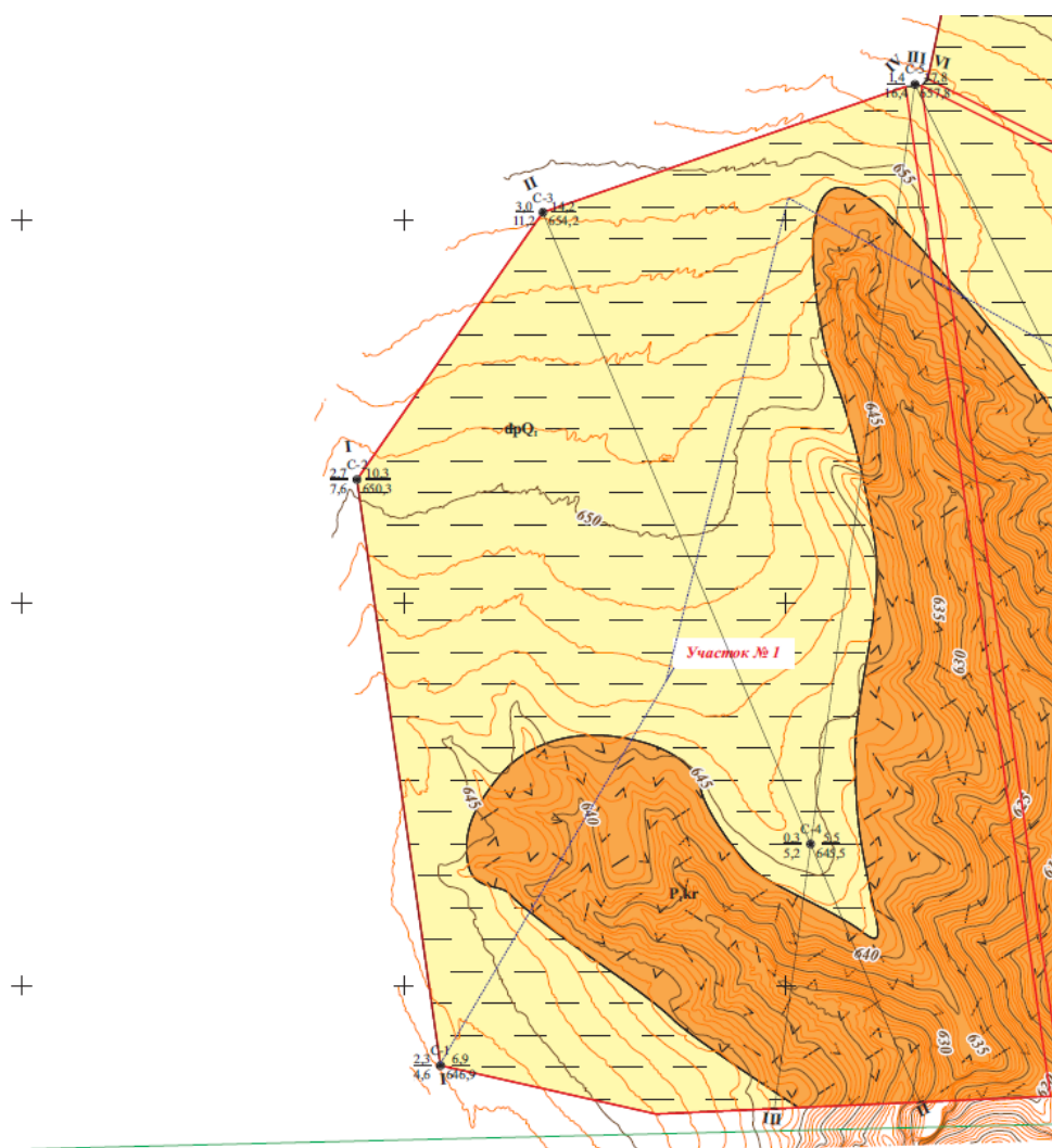
Рис.3.1 Схема геологического строения месторождения «Нура-2 (участок №1)»
