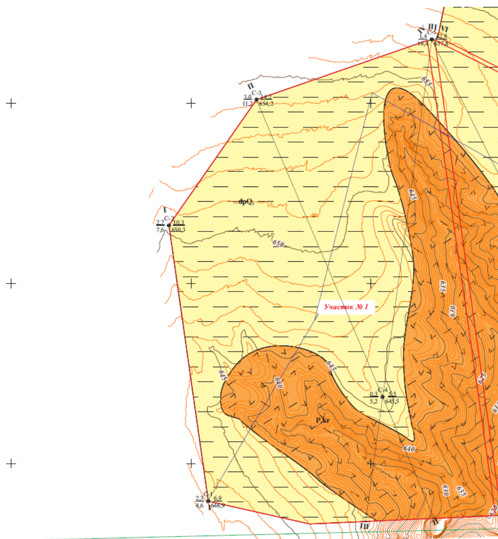
Рис.3.1 Схема геологического строения месторождения «Нура-2 (участок №6)»
