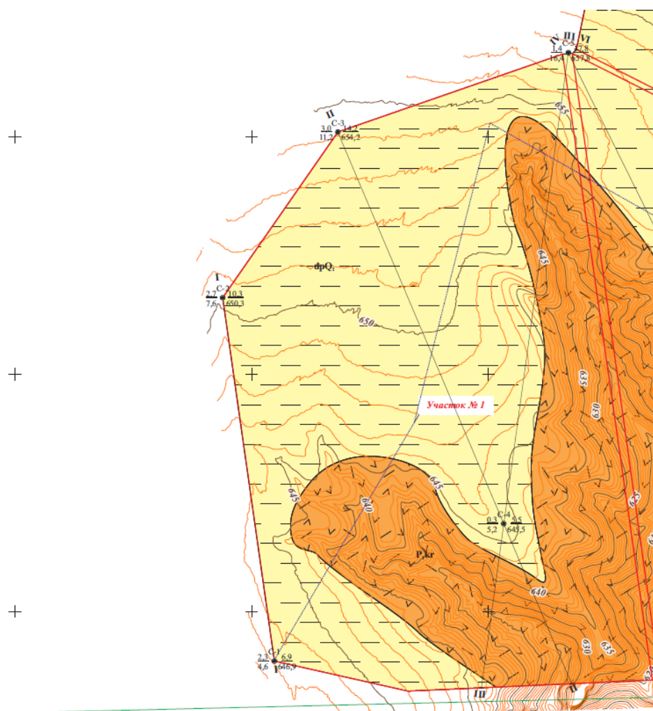
Рис.3.1 Схема геологического строения месторождения «Нура-2 (участок №7)»
