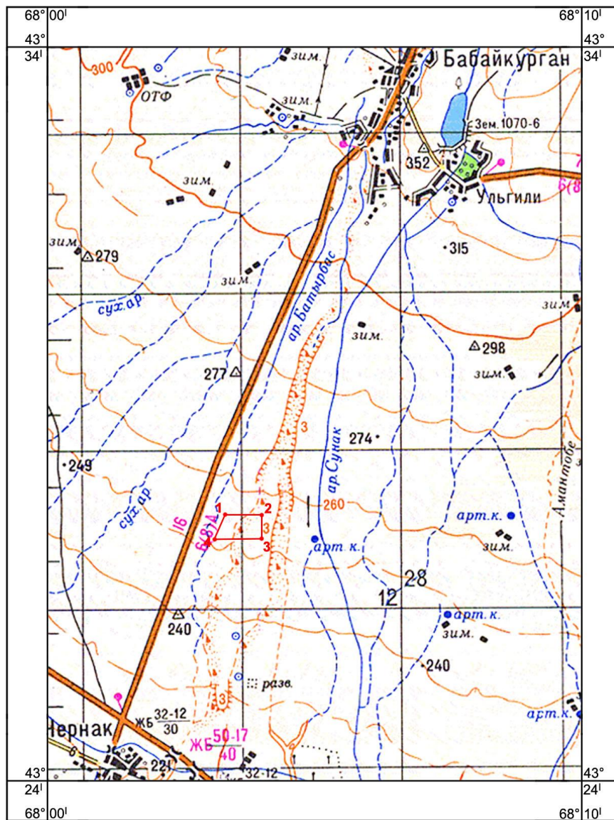
КАРТОГРАММА на добычу песчано-гравийной смеси месторождения Шохан (участок 12) в Сауранском районе Туркестанской области ТОО «Шохан Alem Kaz» Масштаб 1:100 000
