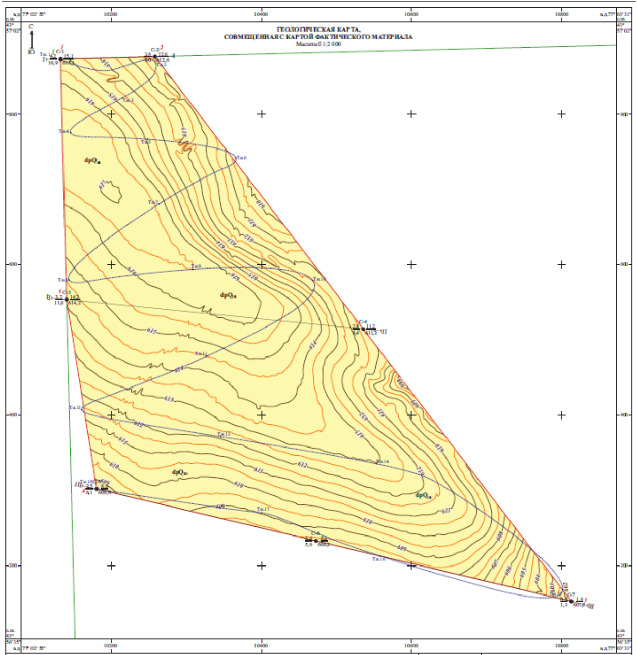
Рис.3.1 Схема геологического строения месторождения «Капшагай-Тас»
