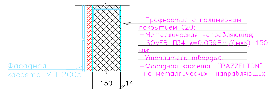
Узел конструкции стен (сэндвич-панели поэлементной сборки)
