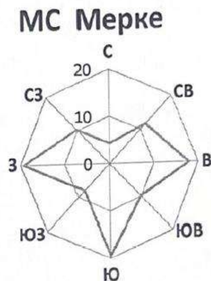
Рисунок 2.1 – Среднегодовая роза ветров района расположения рассматриваемой территории
