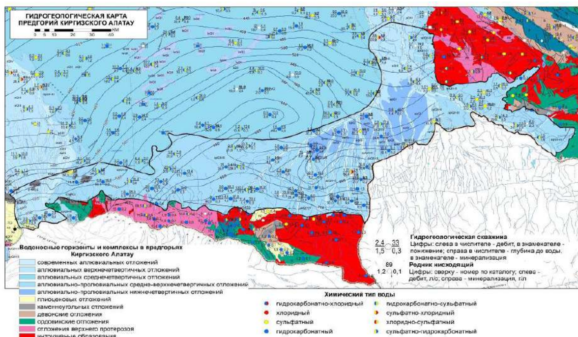
Рисунок 3.1.2 – Схематическая гидрогеологическая карта
