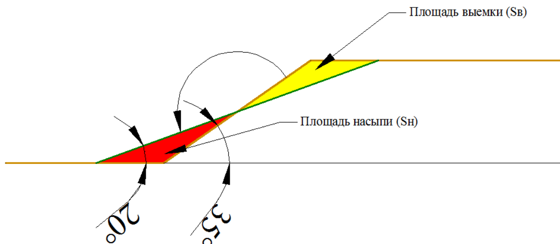
Рис. 1 – Схема выполаживания бортов карьера
