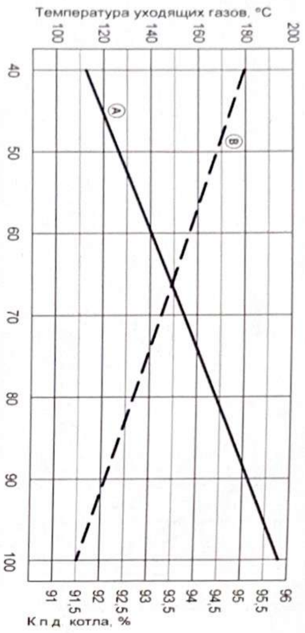
Тепловая мощность водогрейного котла в % от номинальной тепловой мощности
