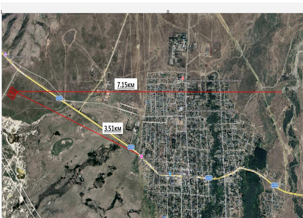
Рисунок 1.1 Ситуационная схема расположения вахтового поселка и бетоносмесительной установки
