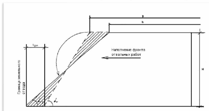
Рис.6. Схема неполаживания карьера с наполнением отвальным продуктом
