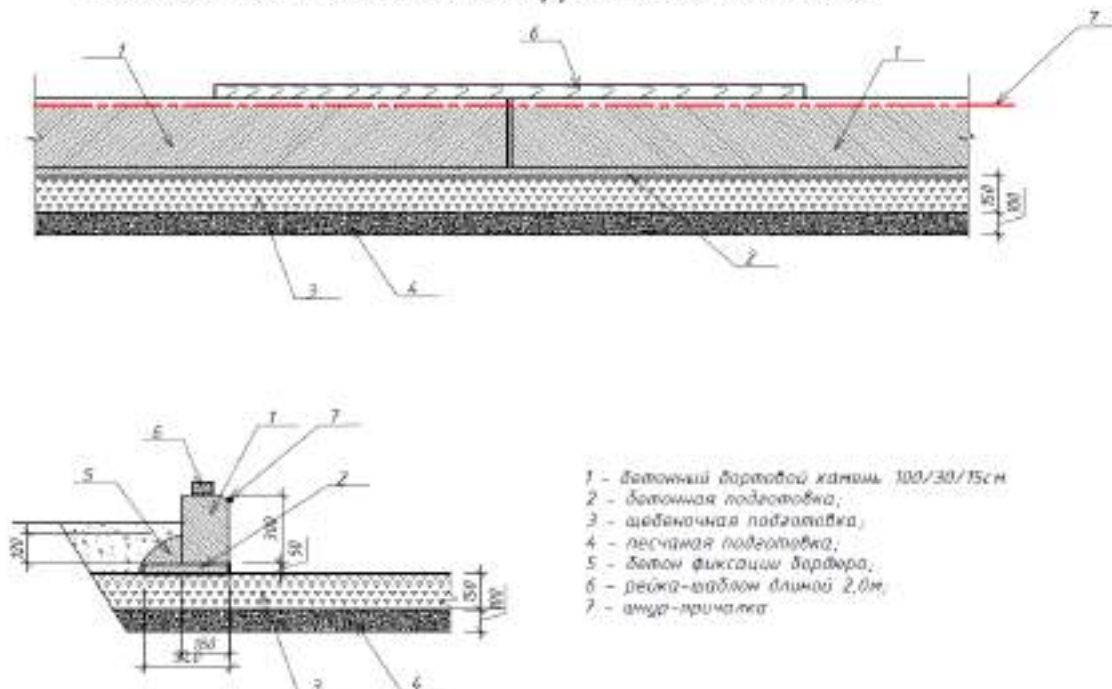
СХЕМА УСТАНОВКИ БОРДЮРНЫХ КАМНЕЙ
