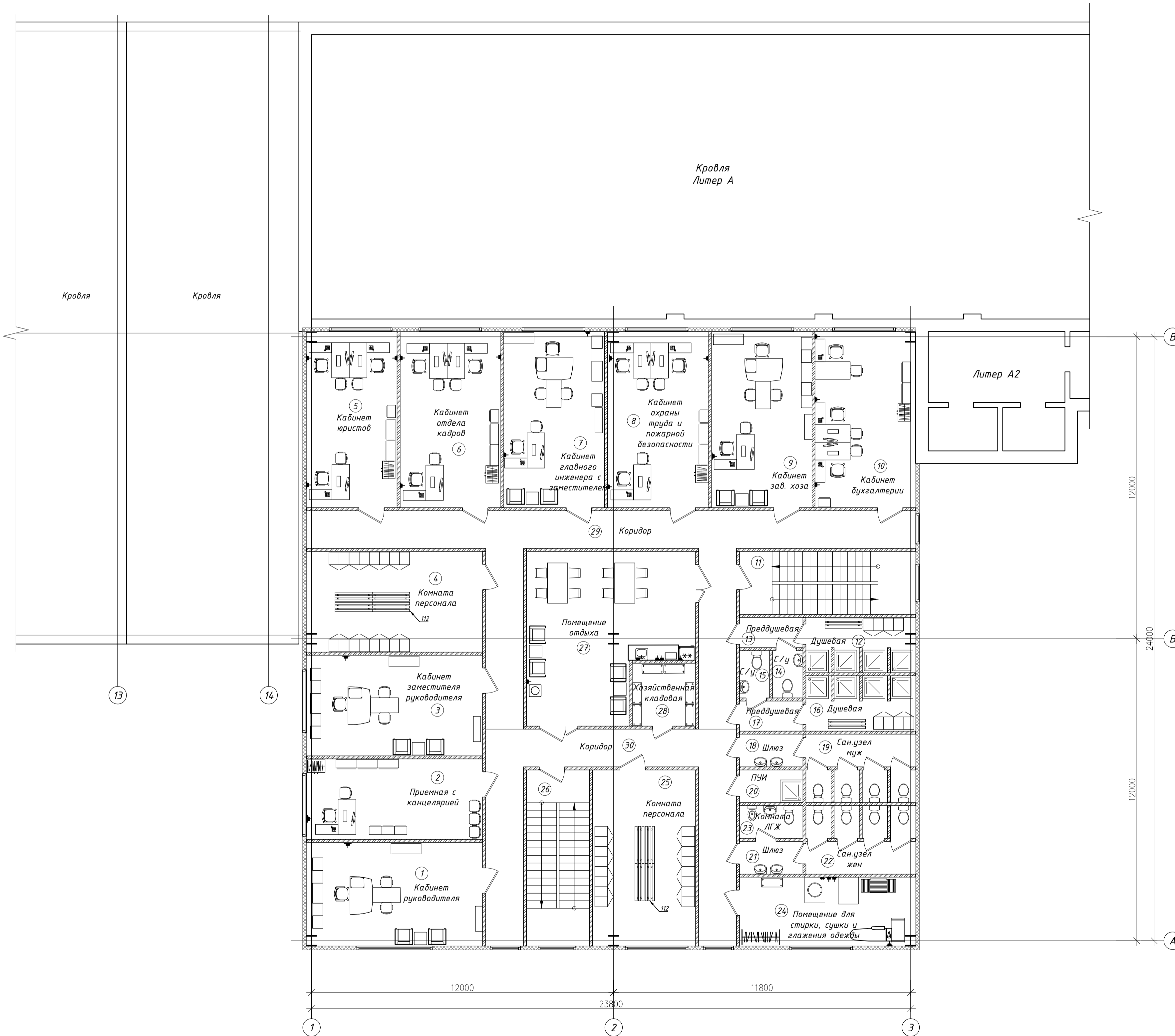
План 2 этажа на отм. +4.200 масштаб 1:100
