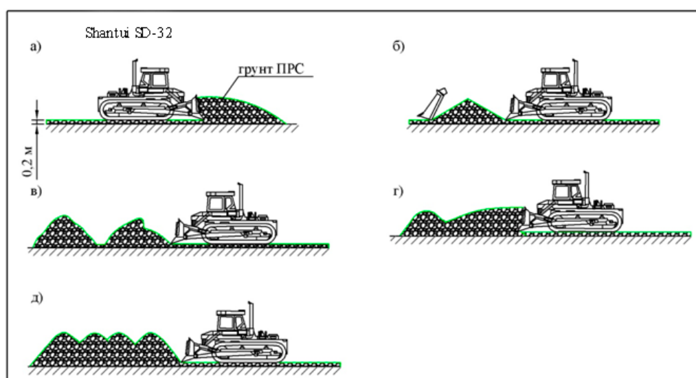
Рис.5.2 Схема планировки и укладки ПРС
