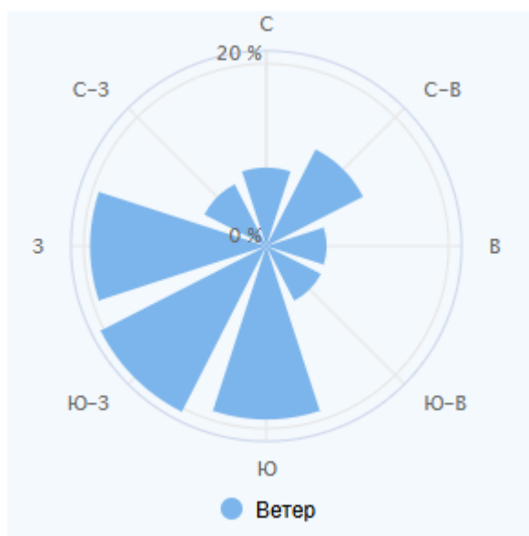
Рис. 3.1 Роза ветров
