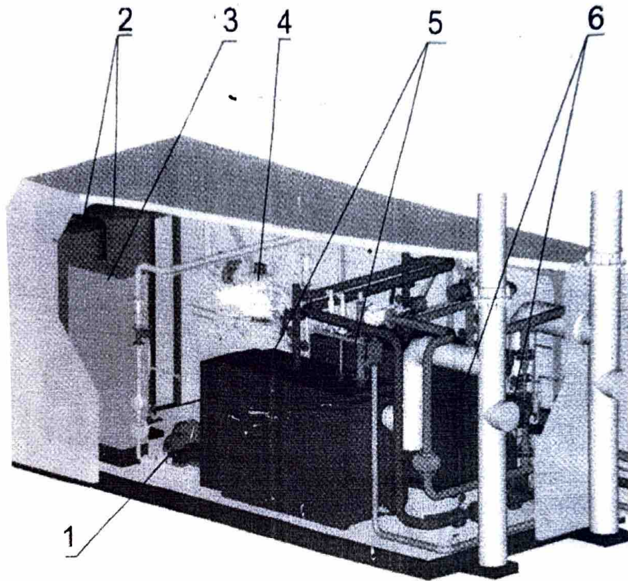
Рисунок 1. Модульная котельная в базовом исполнении
