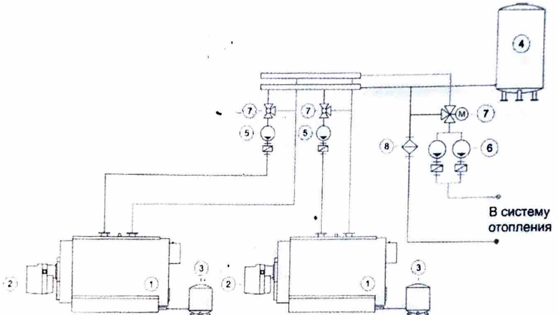
Рисунок 2. Тепловая схема базовой модульной котельной
