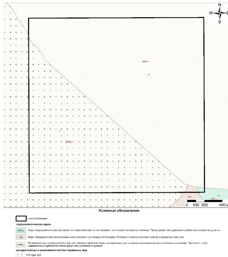
Рисунок 4. Гидрогеологическая карта района месторождения
