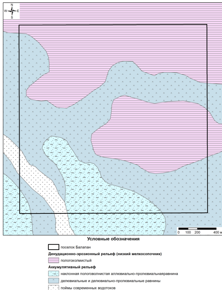
Рисунок 3. Геоморфологическая схема района обследования
