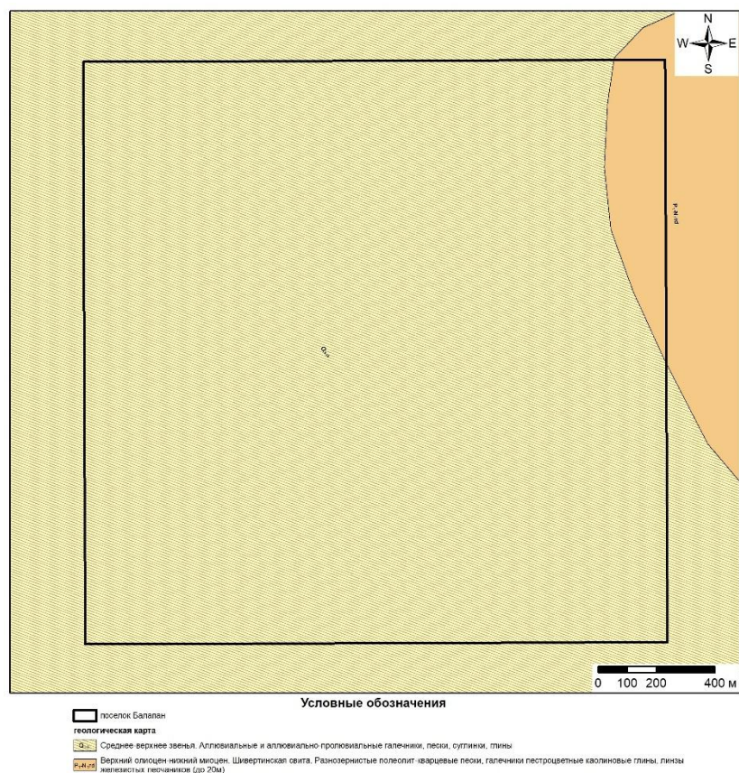
Рисунок 6. Геологическая карта района обследования
