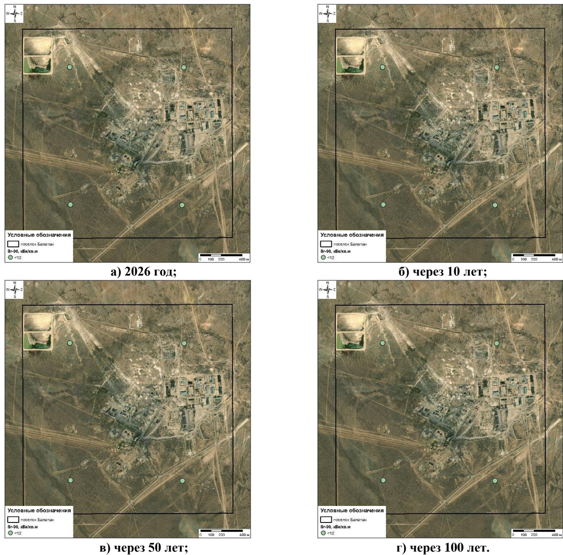
Рисунок 31. Распределение площадной активности ^{90}\text{Sr} в почве
