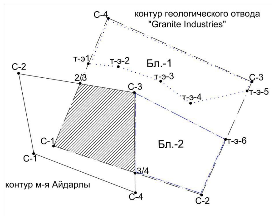
Рис. 1.1 совмещение площадей м-я «Айдарлы» и геологического отвода разведки Бл.-1 – залежь массива гранитов месторождения «Айдарлы-1» Бл.-2 – залежь массива габбро-диабазов месторождения «Айдарлы-2»
