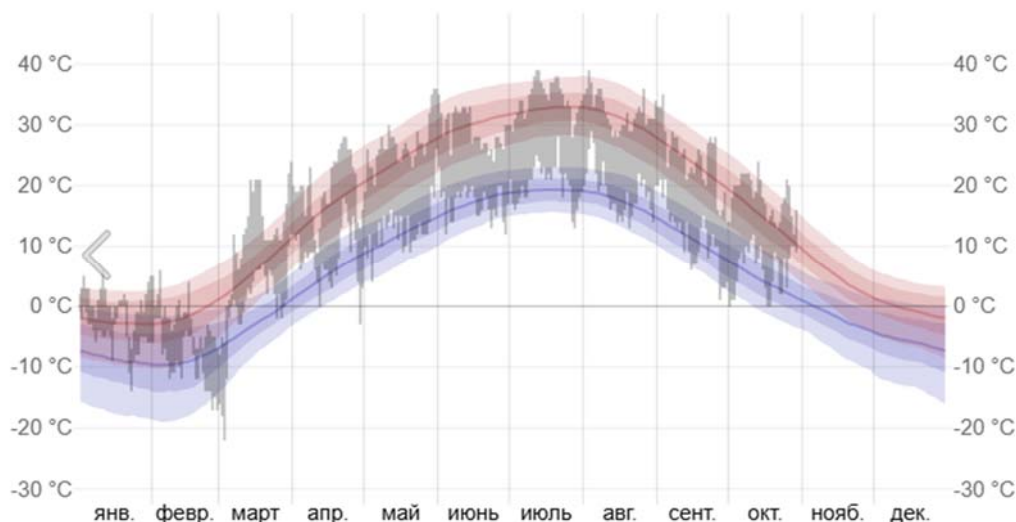
Рисунок 1.1-1. Средняя максимальная и минимальная температура
