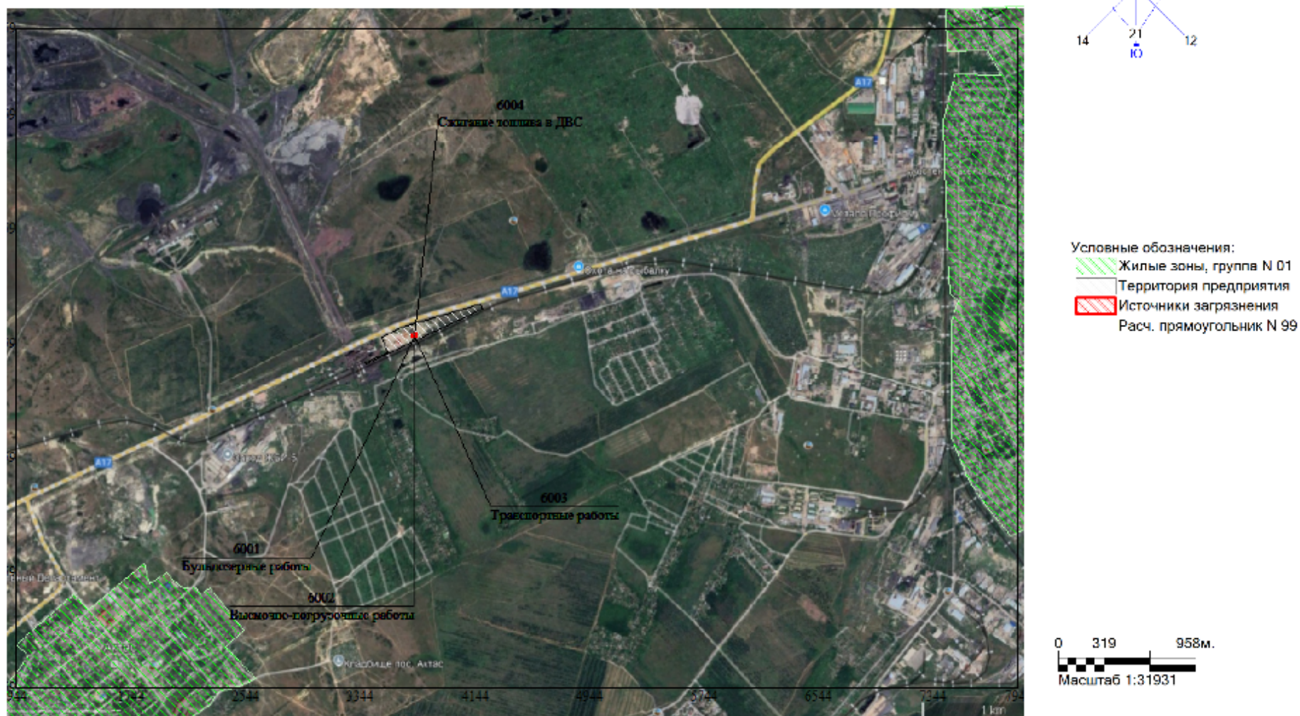
Рисунок 2.1 – Масштабная карта-схема с источниками выбросов загрязняющих веществ в атмосферу
