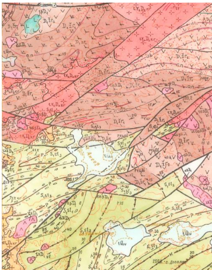
Рисунок 4. Геологическая карта участка работ
