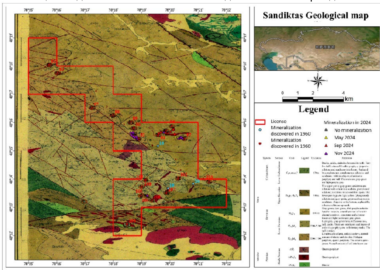
Рисунок 5. Геологическая карта участка Сандыктас
