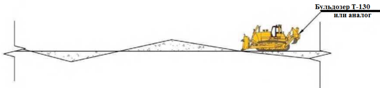
Рис.5.3 Технологическая схема планировки
