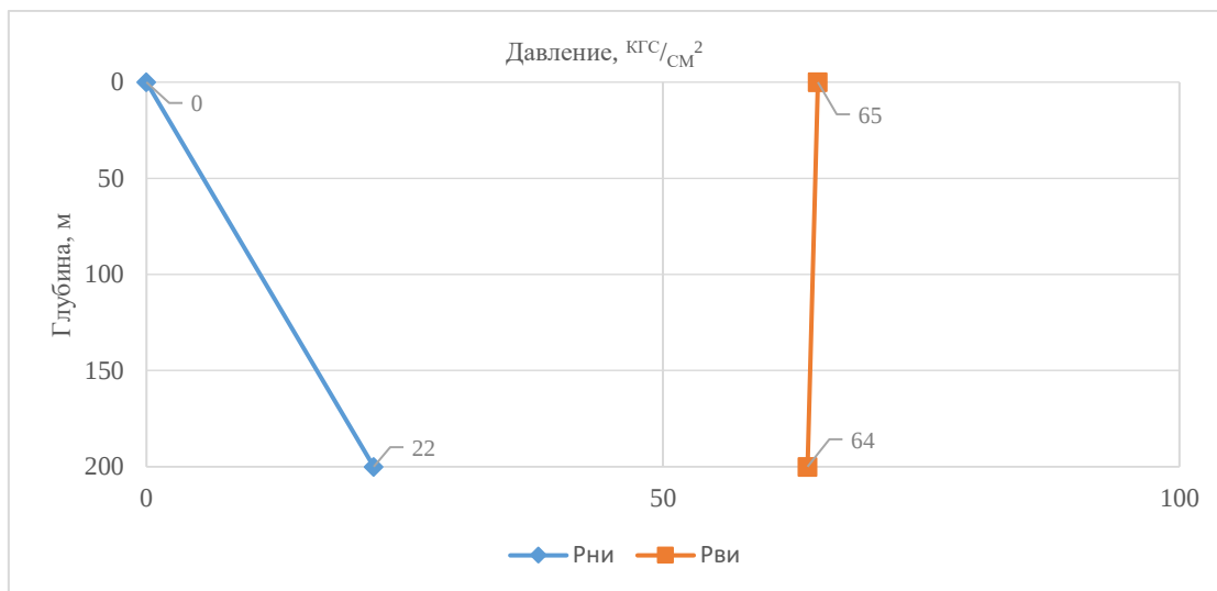
Рисунок 9.1 – Распределение избыточных внутренних и наружных давлений по длине колонны Ø 426 мм (кондуктор)
