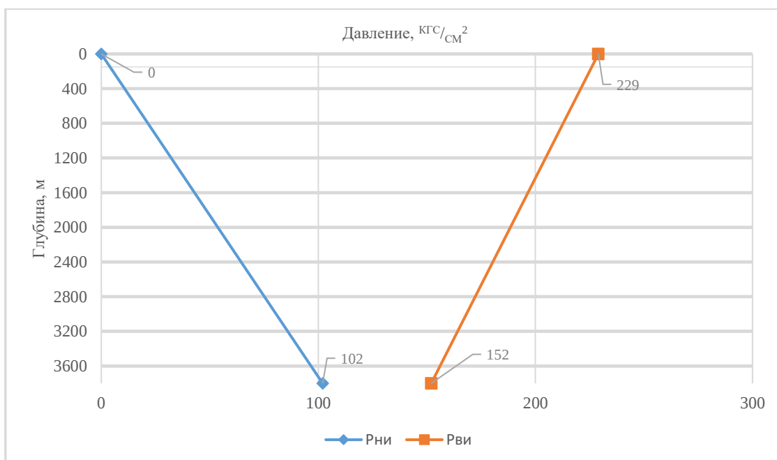
Рисунок 9.4 – Распределение избыточных внутренних и наружных давлений по длине колонны Ø 168,3 мм (эксплуатационная колонна)
