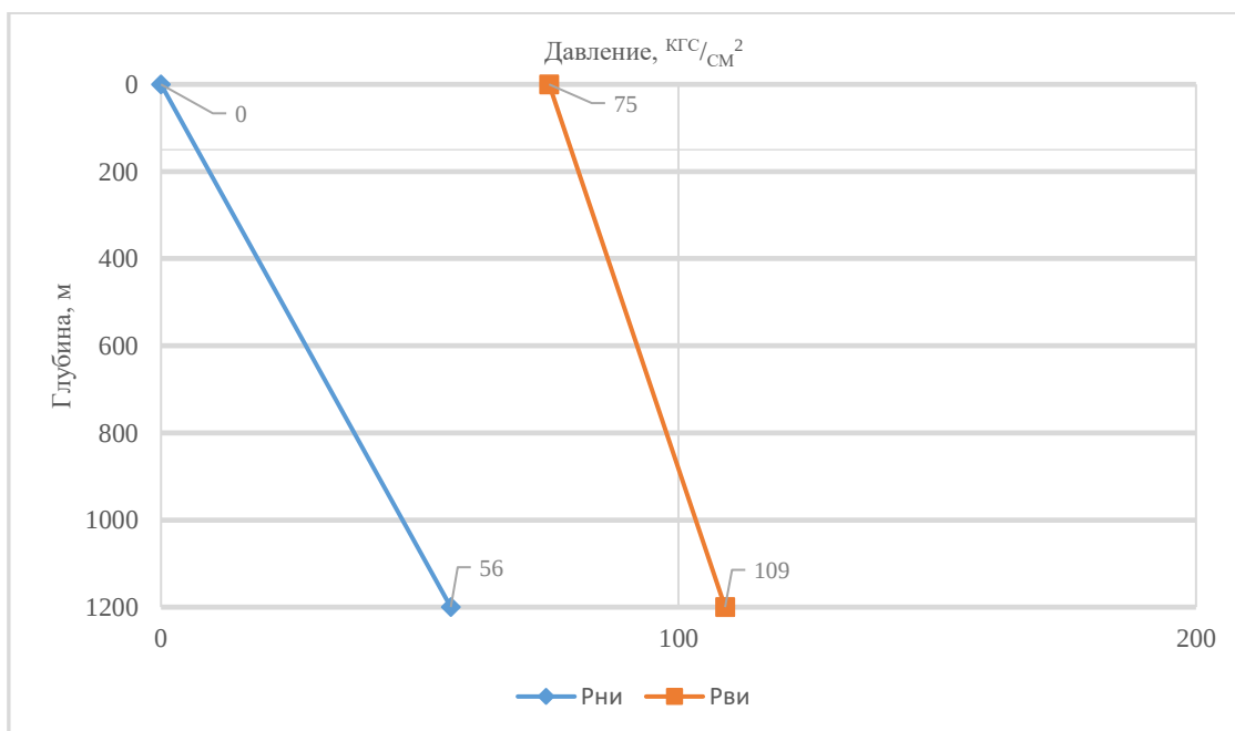
Рисунок 9.2 – Распределение избыточных внутренних и наружных давлений по длине колонны Ø 324 мм (1 промежуточная колонна)
