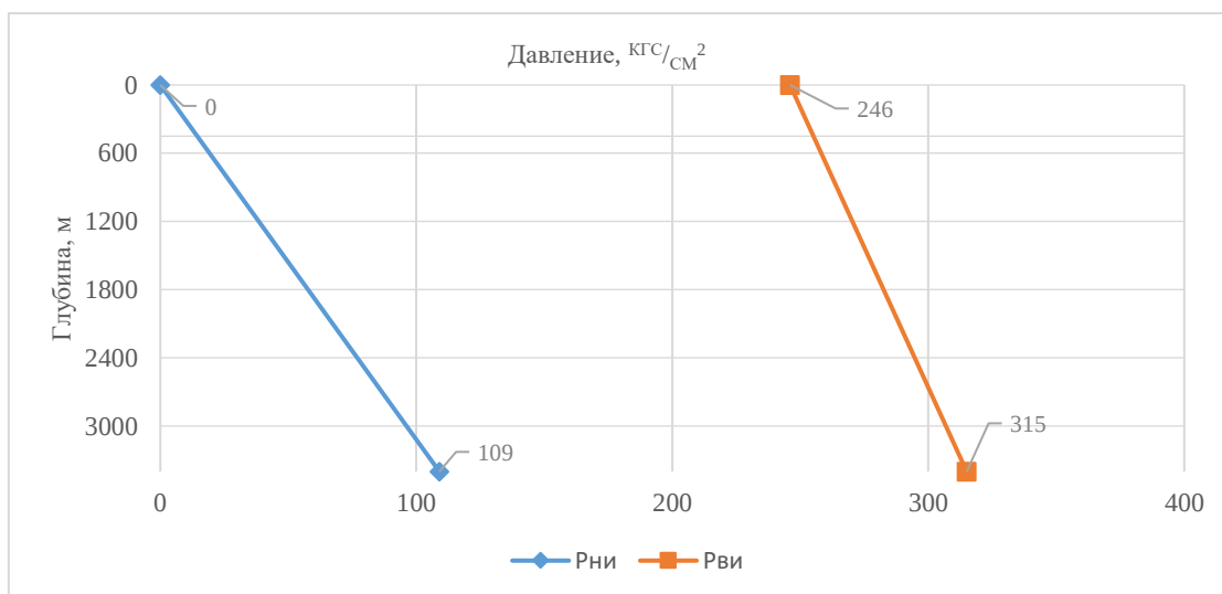
Рисунок 9.3 – Распределение избыточных внутренних и наружных давлений по длине колонны Ø 244,5 мм (2 промежуточная колонна)
