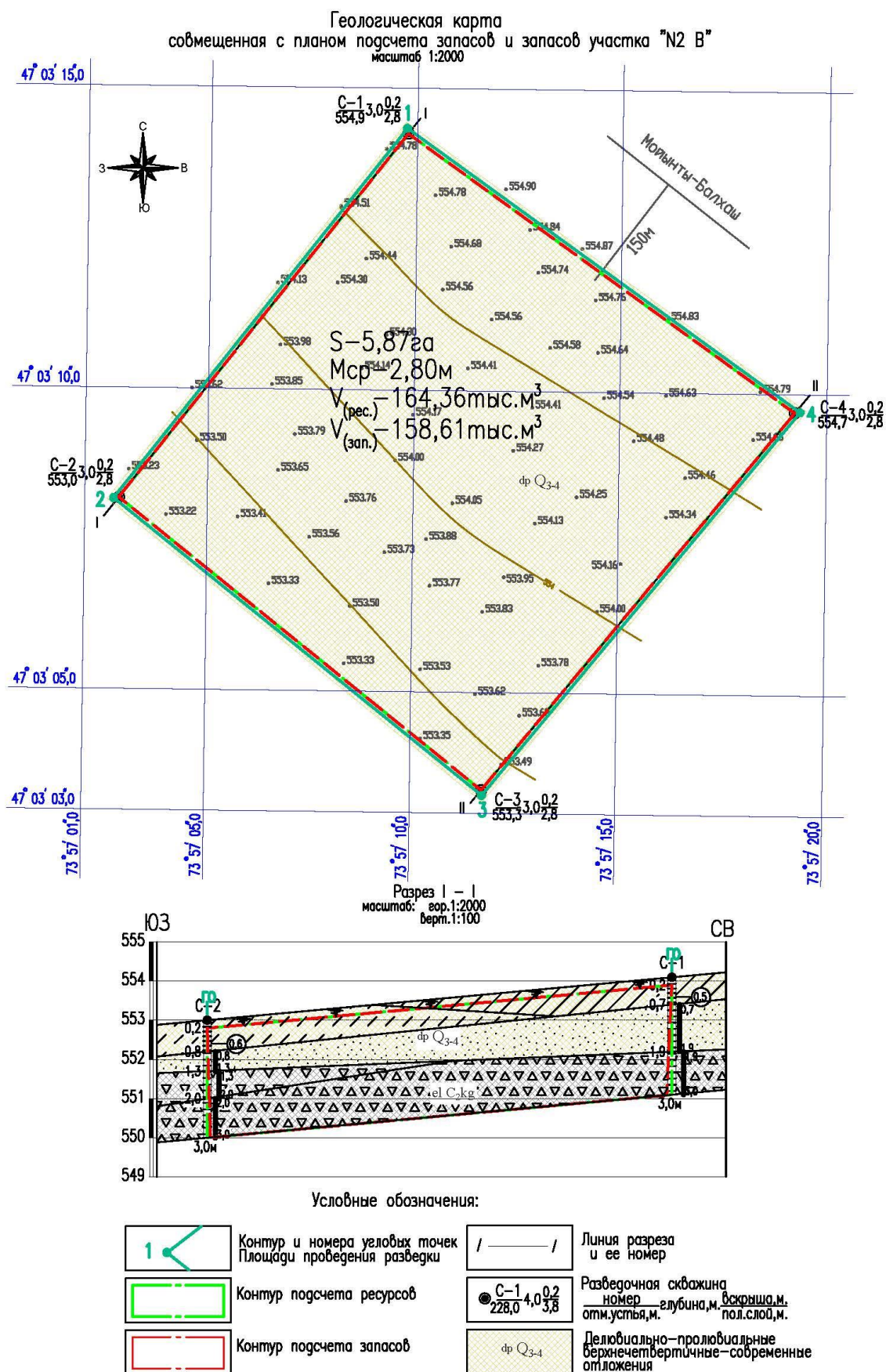
Рис. 2.6 Схема геологического строения участка №2В
