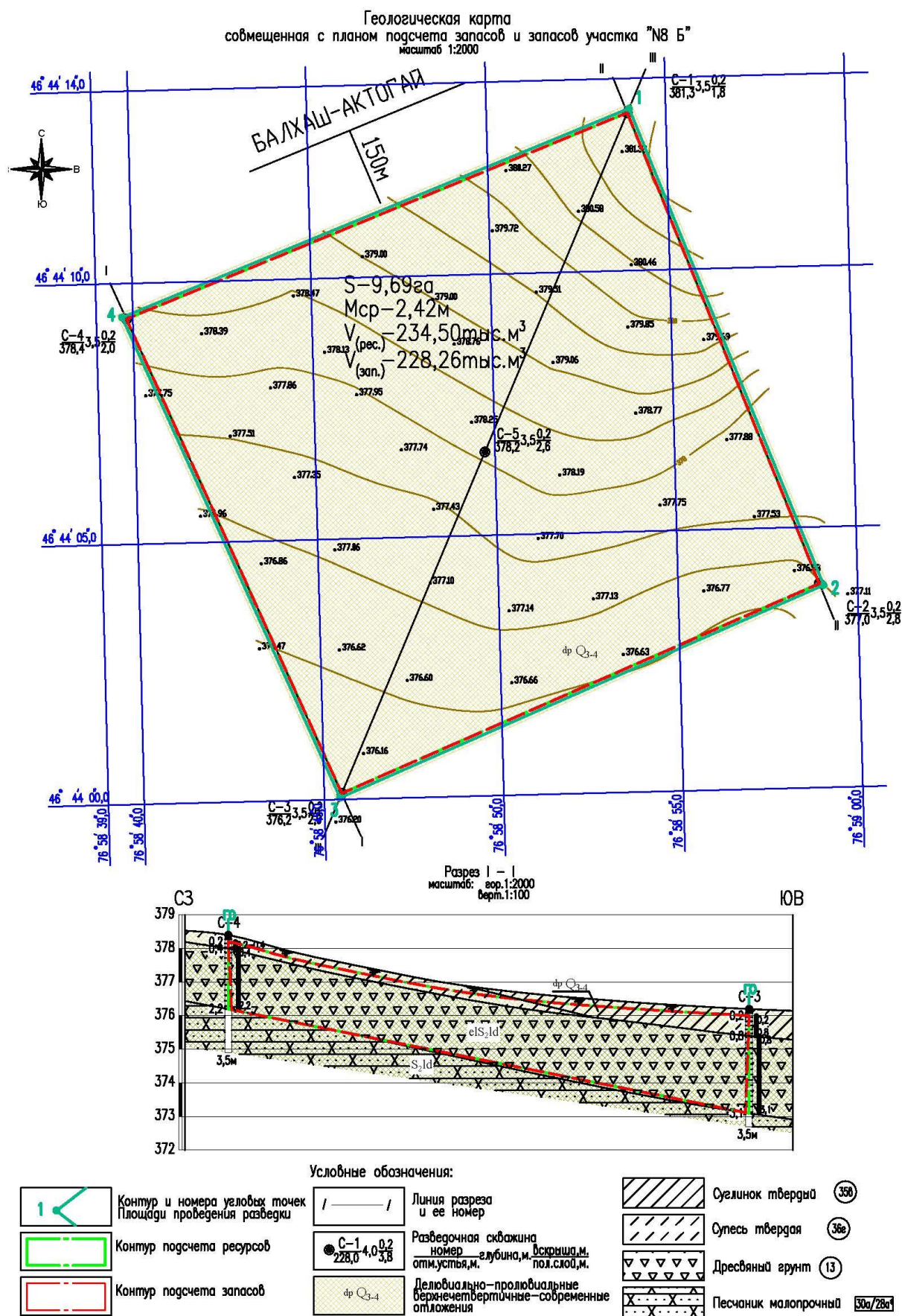
Рис. 2.10. Схема геологического строения участка №8Б.
