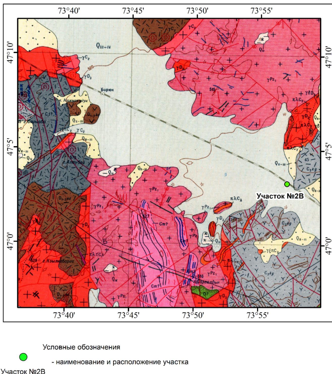
Рис.2.1 Геологическая карта расположения участка №2В(выкопировка из геологической карты листа L-43-VIII) масштаб 1:200 000
