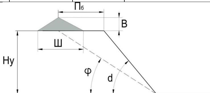
Рис.3.1 Схема уступа
