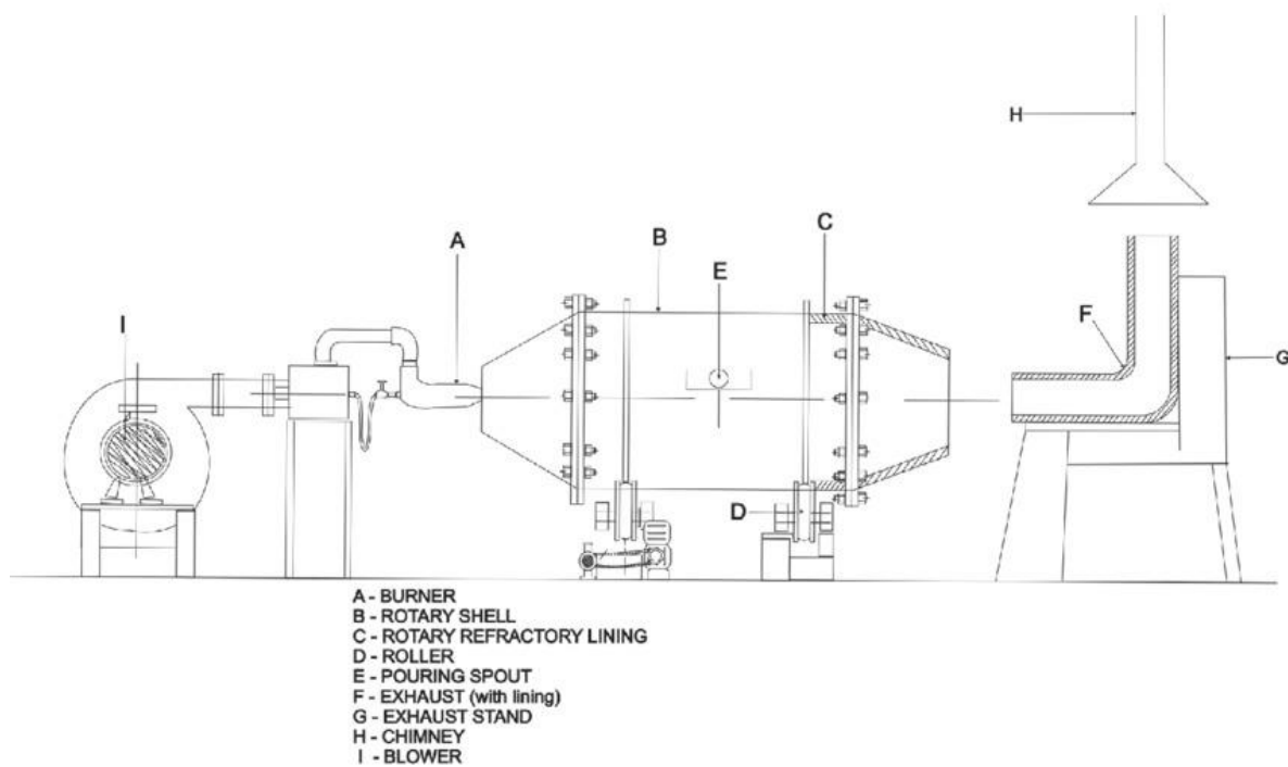
Схема 1. Роторный печь
